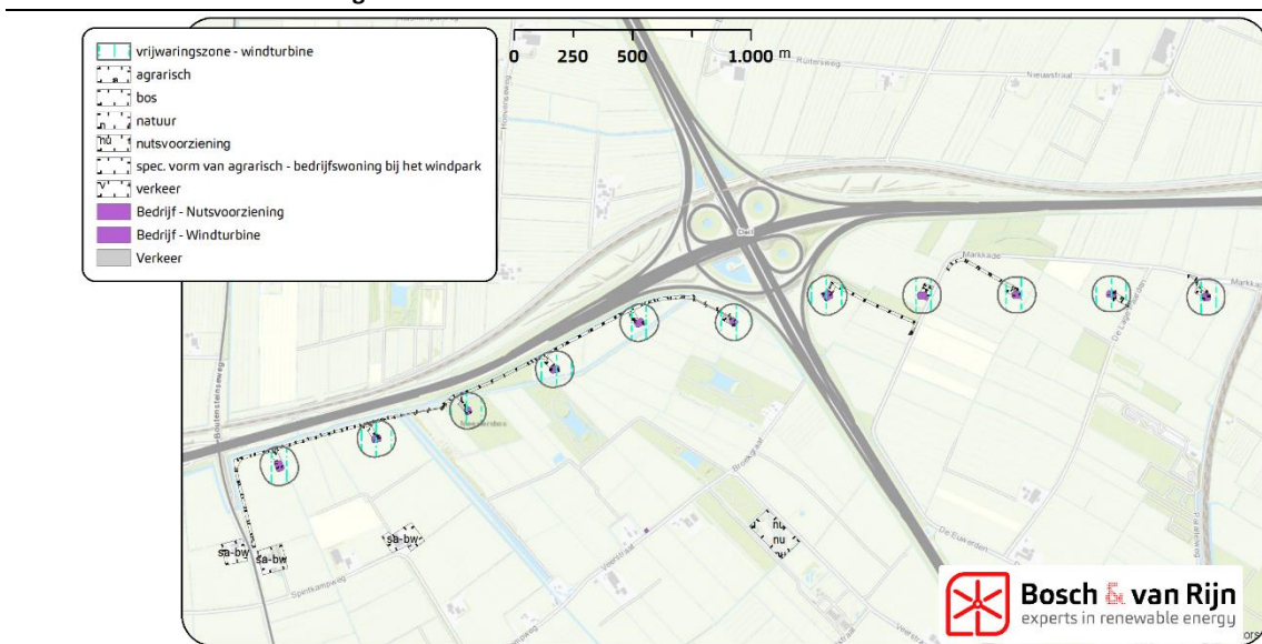
Figuur 7 Concept plankaart, waarop de fundering van de windturbines binnen de paarse vlakken moet blijven. Dit laat enige schuifruimte toe.
