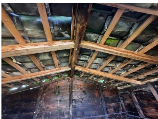
Figuur 5.4: geen dakbeschot onder de dakpannen
