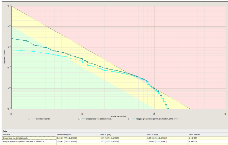
Grafiek 4.3: fN-curve berekend groepsrisico toekomstige situatie, 315 evenementen
