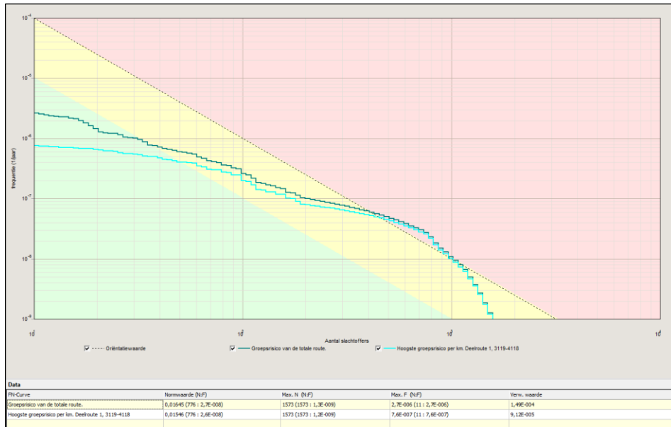
Grafiek 4.2: fN-curve berekend groepsrisico toekomstige situatie, 365 evenementen
