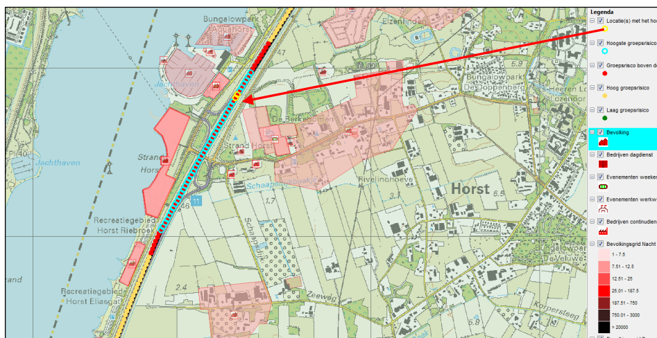
Figuur 4.2: locatie met hoogste GR weg-toekomstige situatie
