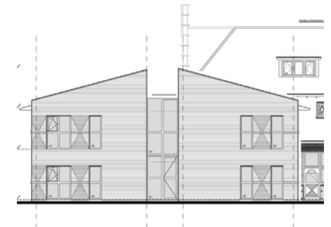
Afb. 36b: 't Waeghuys, ontwerp achtergevel (bron: De BRUIN Architecten)
