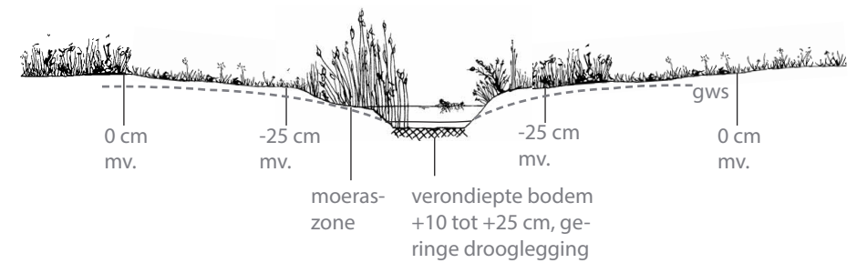
Afb.: Schets voorgenomen ingreep beekloop
