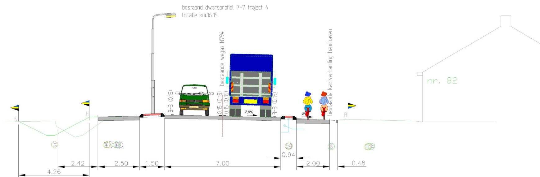
principe dwarsprofiel 7-7 traject 4 locatie km.16.15
