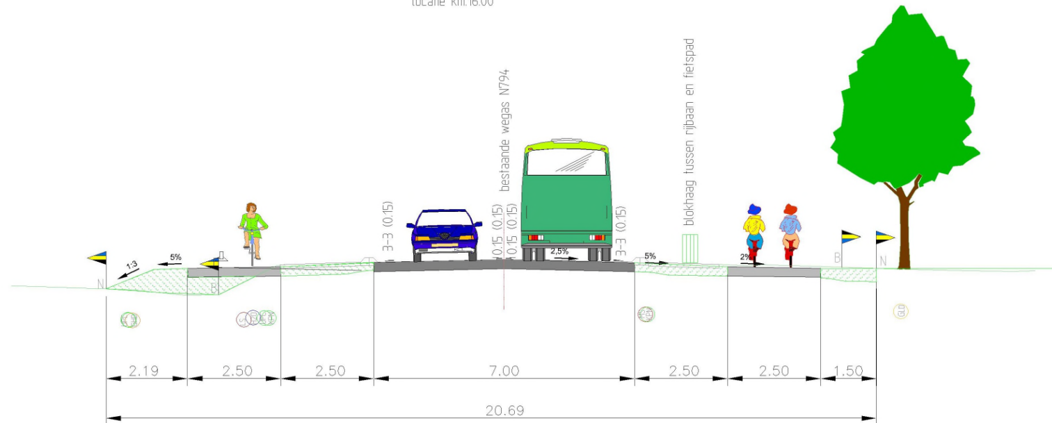
bestaand dwarsprofiel 6-6 traject 3 locatie km.16.00
