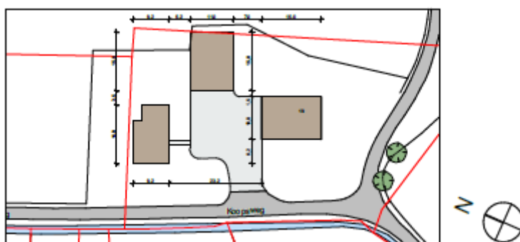
SITUATIE NIEUW schaal 1:500
