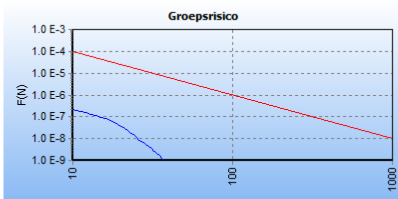
5.1 Figuur 6.1 FN curve voor 8376_leiding-N-570-20-deel-1 van N.V. Nederlandse Gasunie voor de kilometer tussen stationing 2180.00 en stationing 3180.00
