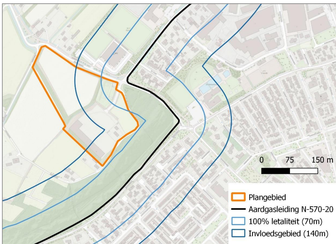
Figuur 2. Invloedsgebied en 100%-letaliteitscontour van aardgasleiding N-570-20
