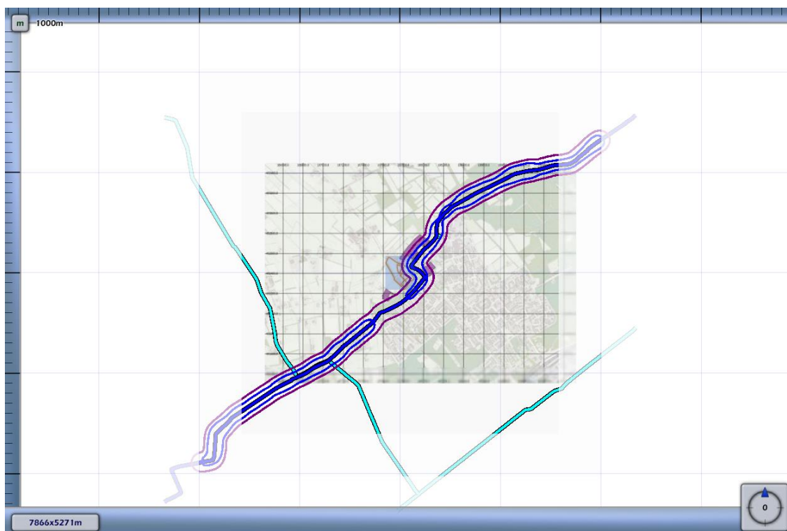
3.1 Figuur 3.1 Plaatsgebonden risico voor 6706_leiding-N-570-20-deel-1 van N.V. Nederlandse Gasunie
