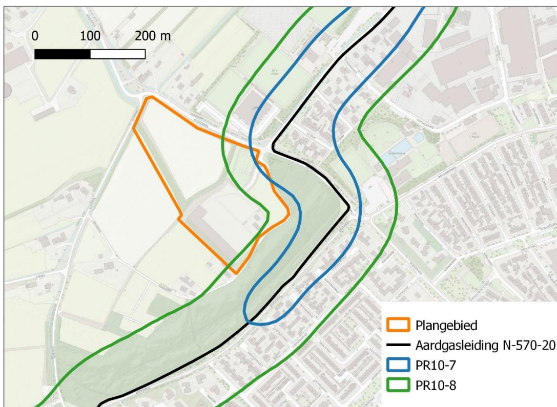
Figuur 3. PR-contouren aardgasleiding N-570-20
