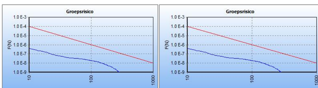
Figuur 4. Groepsrisico N-570-20, huidig (links) en toekomstig (rechts)
