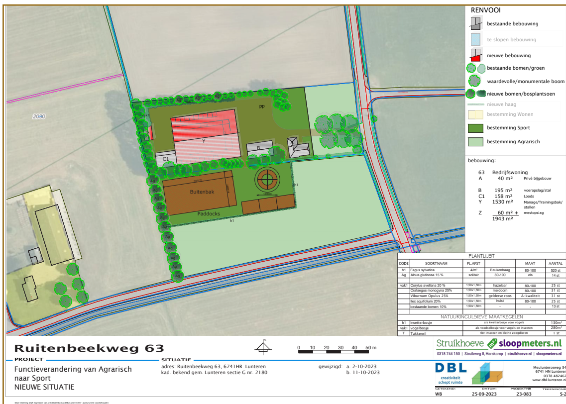
Afbeelding 1.4: Nieuwe situatie. Bron: 23-083, Plattegrond nieuwe situatie DBL, 2023.
