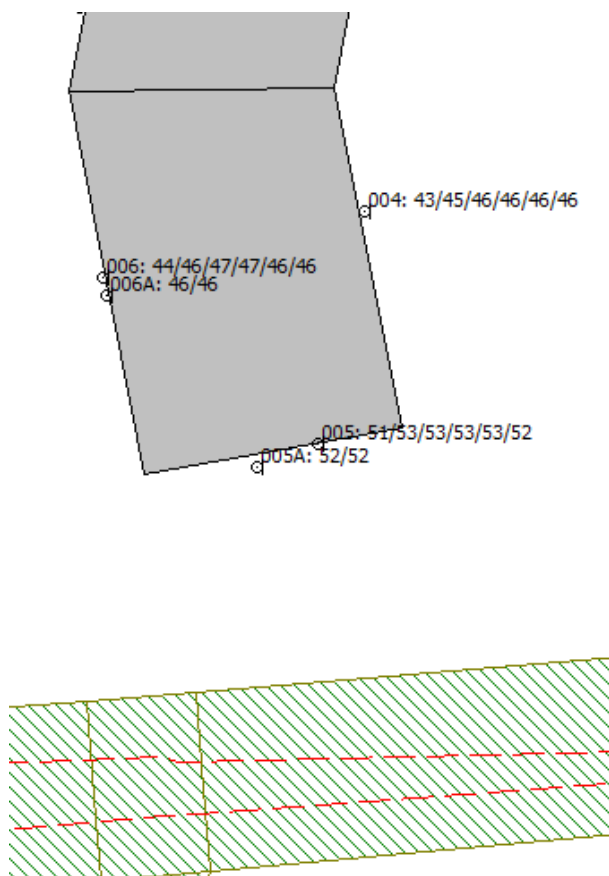
Figuur 3 geluidsbelasting Eikenlaan per gevel inclusief aftrek art. 110g Wgh (5dB)
