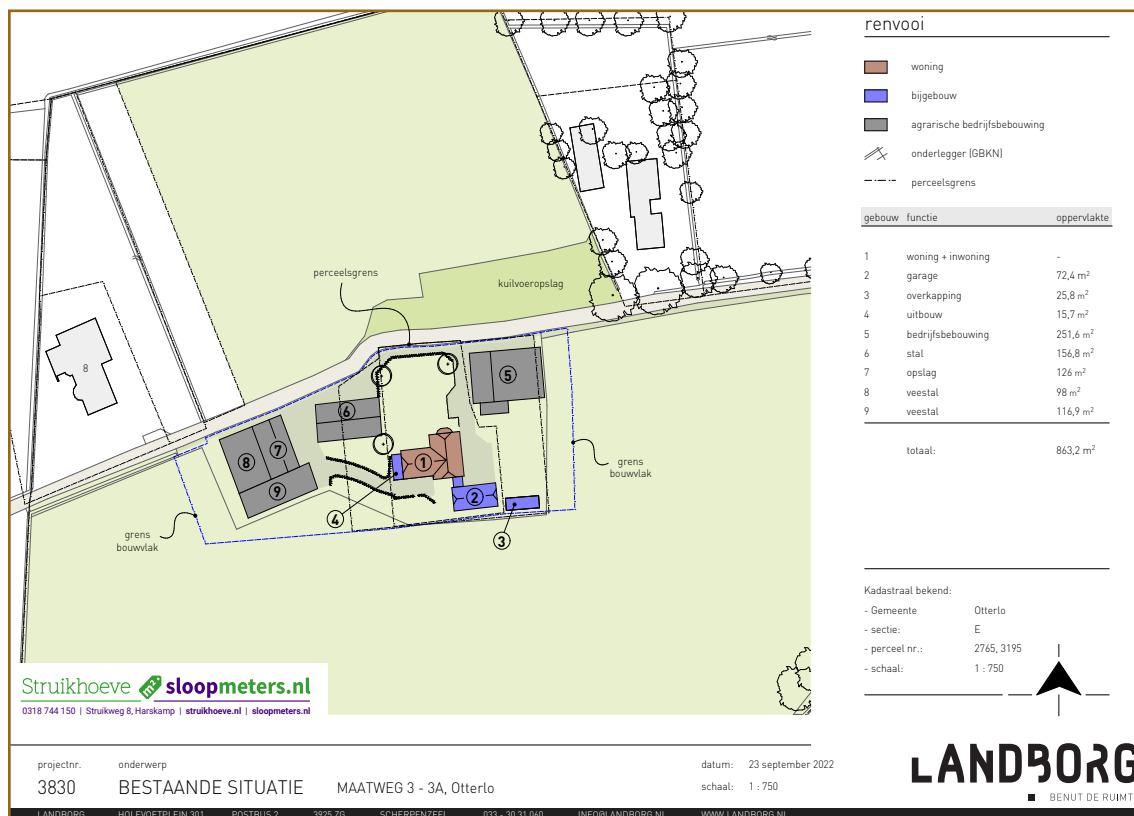
Afb. 1.3: Bestaande situatie. Bron: 3830, bestaande situatie, Landborg, 2022.
