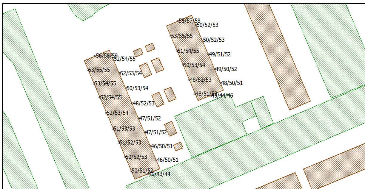
Figuur 11: Cumulatieve geluidsbelasting toekomstige woningen deelgebied 7b (exclusief aftrek).
