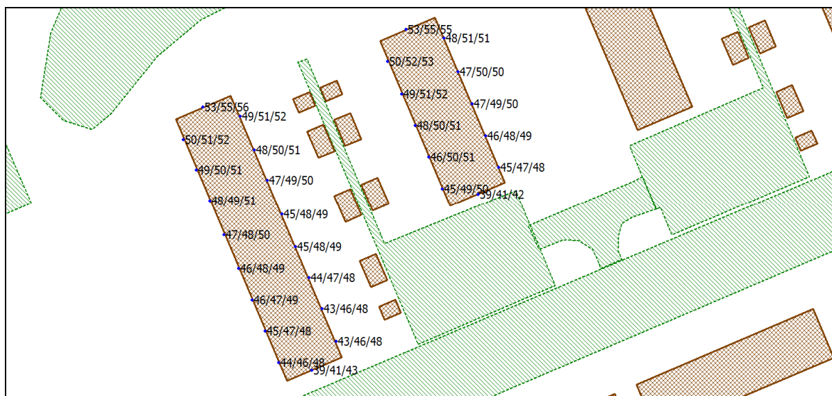
Figuur 6: Geluidsbelasting toekomstige woningen deelgebied 6b (variant 2) vanwege de N224.
