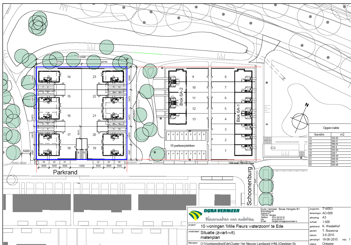
Figuur 1: Matenplan deelgebied 6b volgens variant 1 (8 2/1-kappers en 2 vrijstaande woningen).
