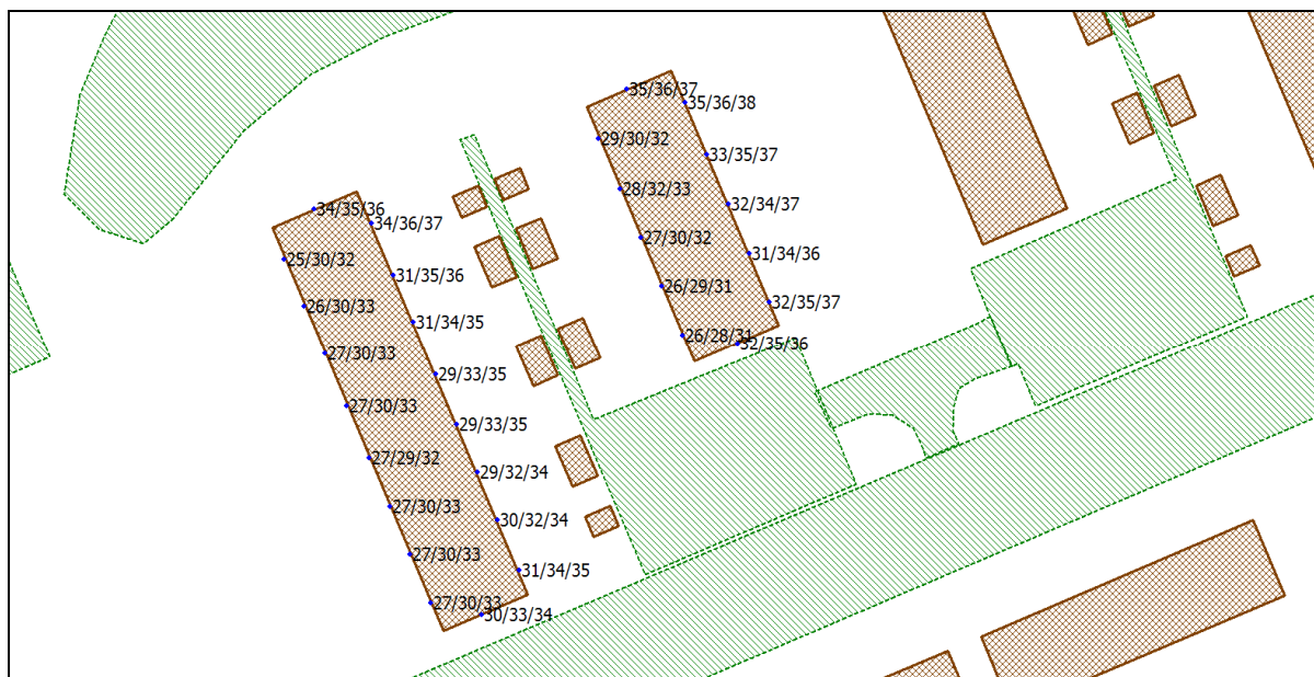
Figuur 7: Geluidsbelasting toekomstige woningen deelgebied 6b (variant 2) vanwege de Proosdijerveldweg.
