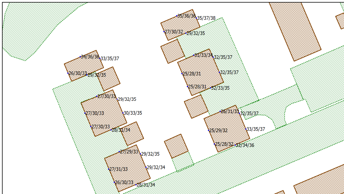
Figuur 5: Geluidsbelasting toekomstige woningen deelgebied 6b (variant 1) vanwege de Proosdijerveldweg.
