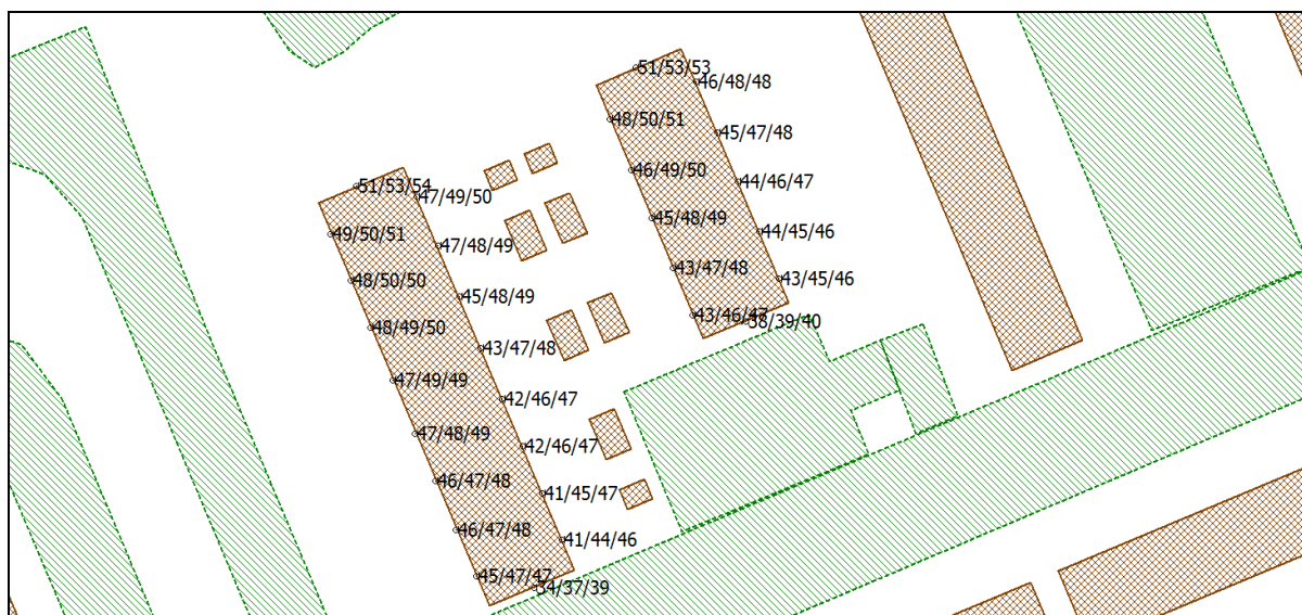
Figuur 8: Geluidsbelasting toekomstige woningen deelgebied 7b vanwege de N224.
