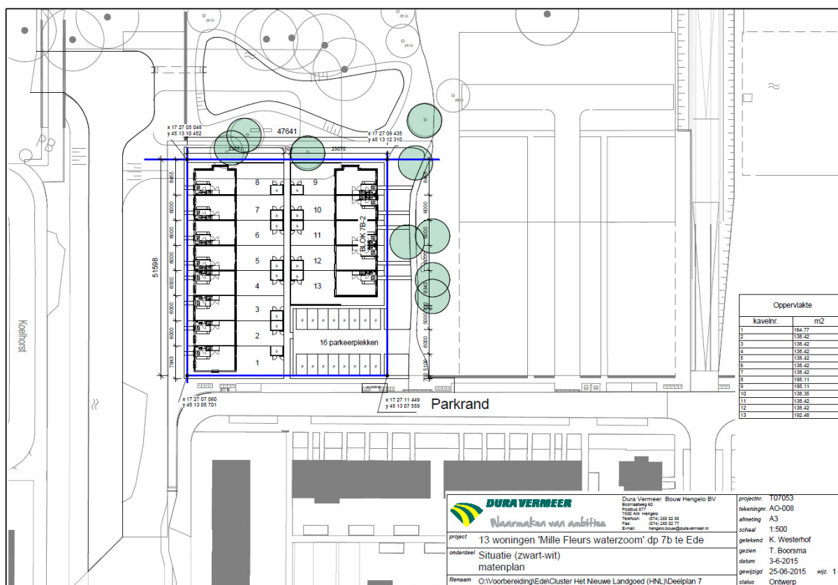
Figuur 3: Matenplan deelgebied 7b (13 rijwoningen).
