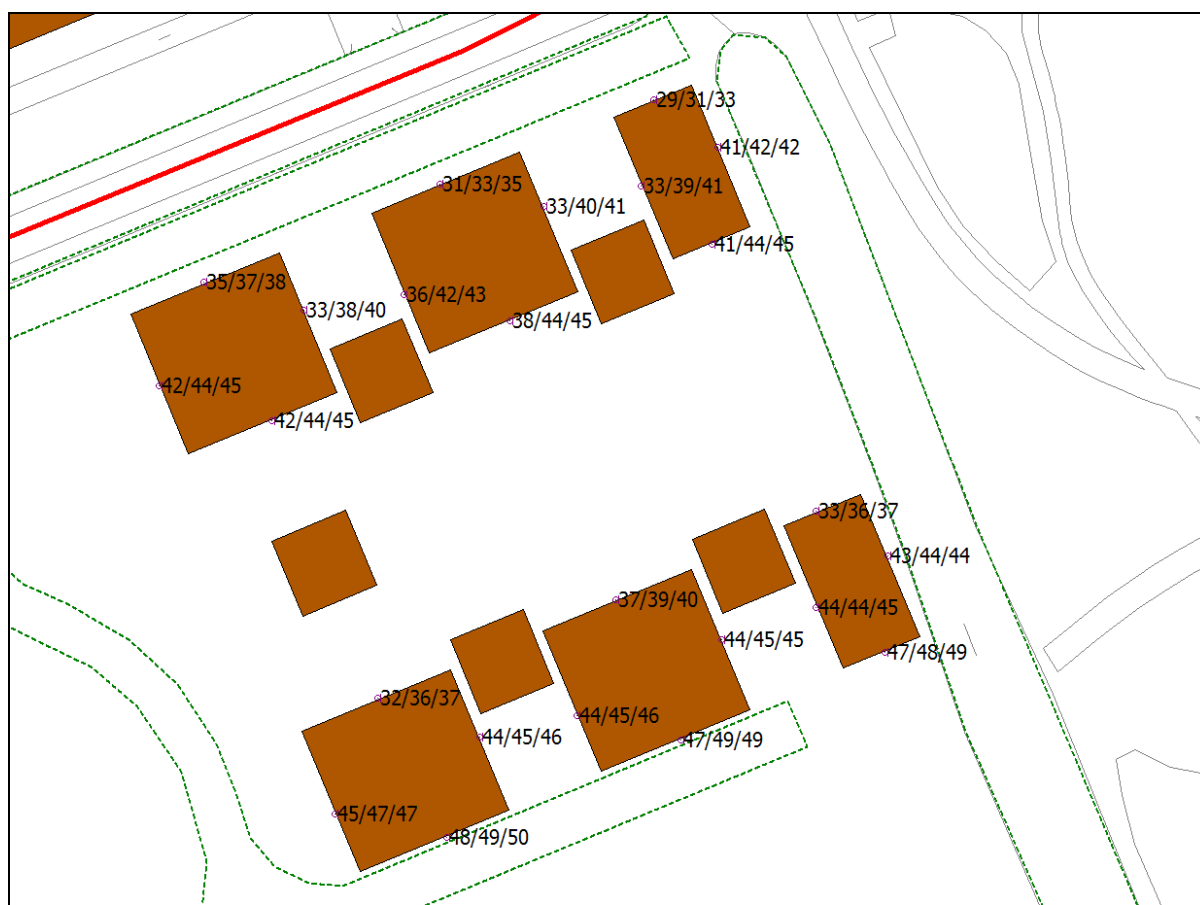
Figuur 2: Geluidsbelasting toekomstige woningen vanwege de N224.
