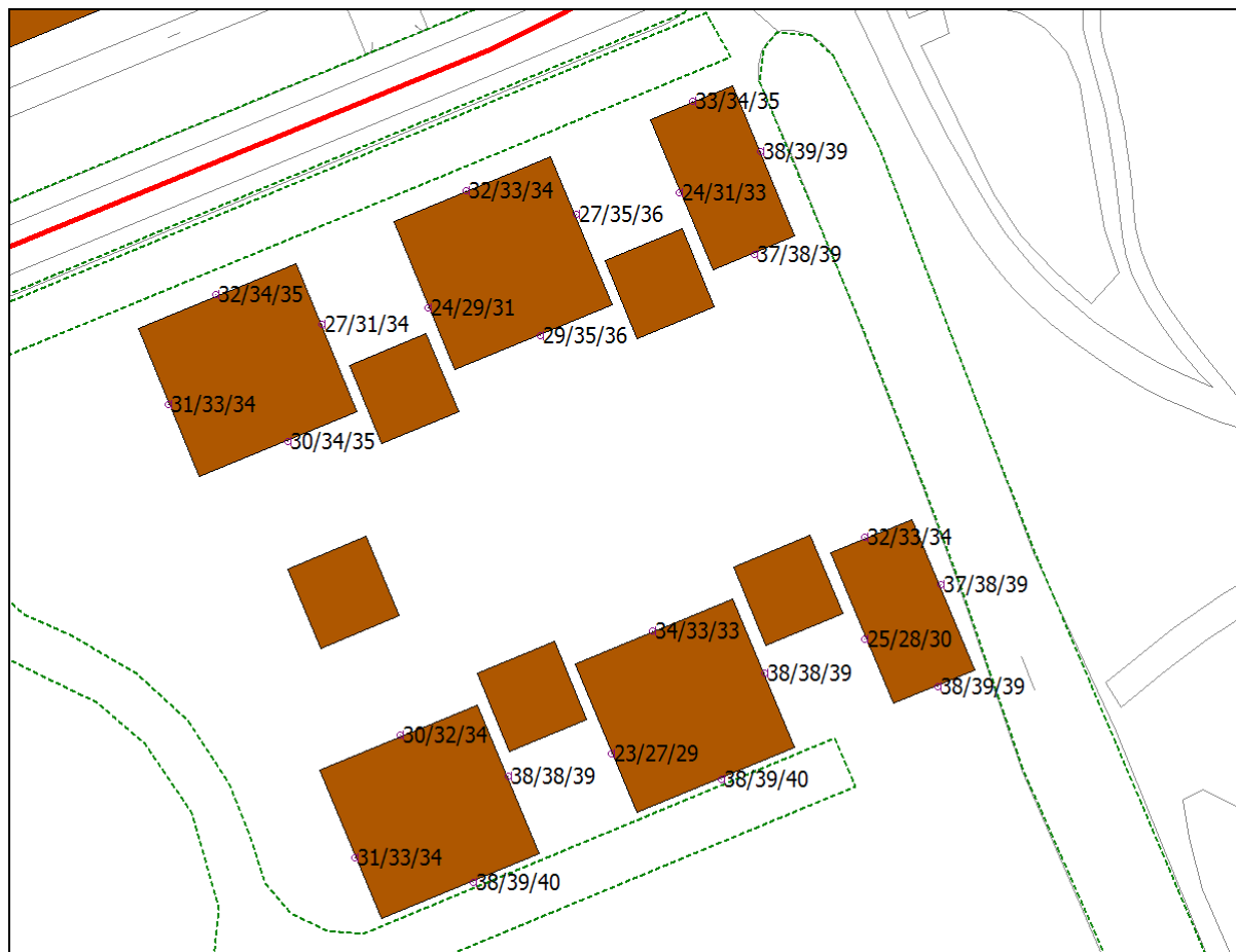
Figuur 3: Geluidsbelasting toekomstige woningen vanwege de Lunterseweg.
