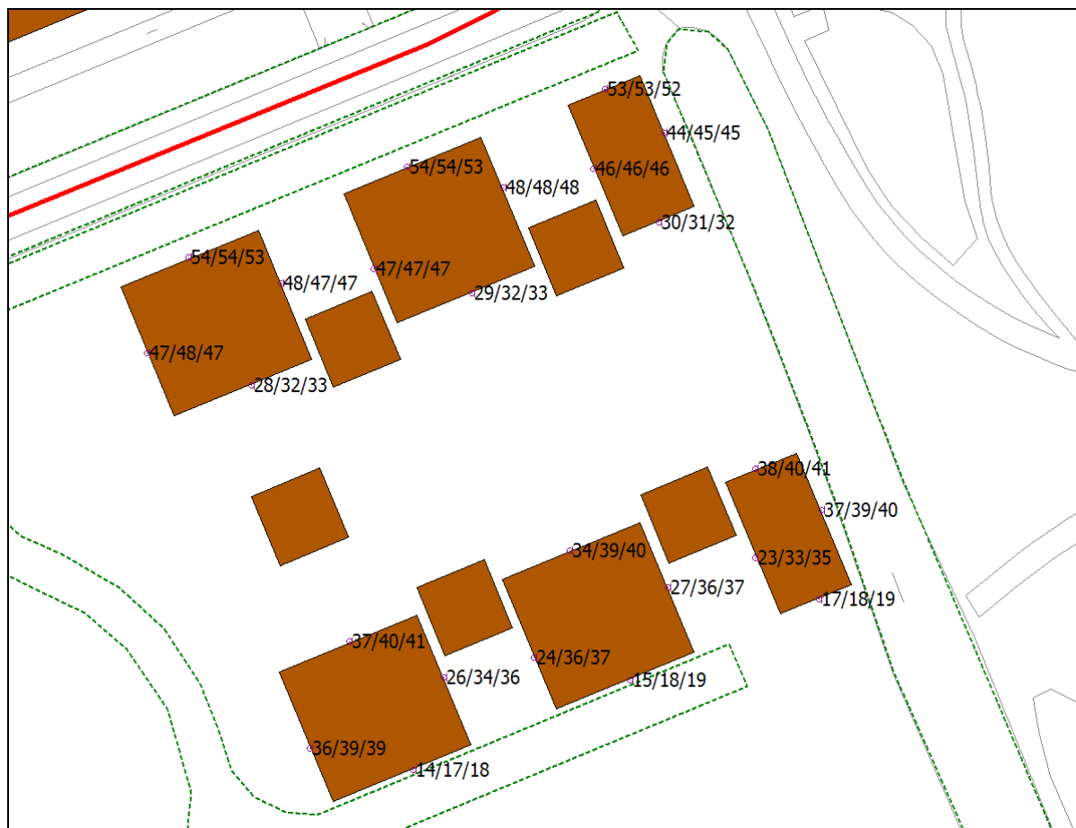
Figuur 4: Geluidsbelasting toekomstige woningen vanwege de Stakenberg.
