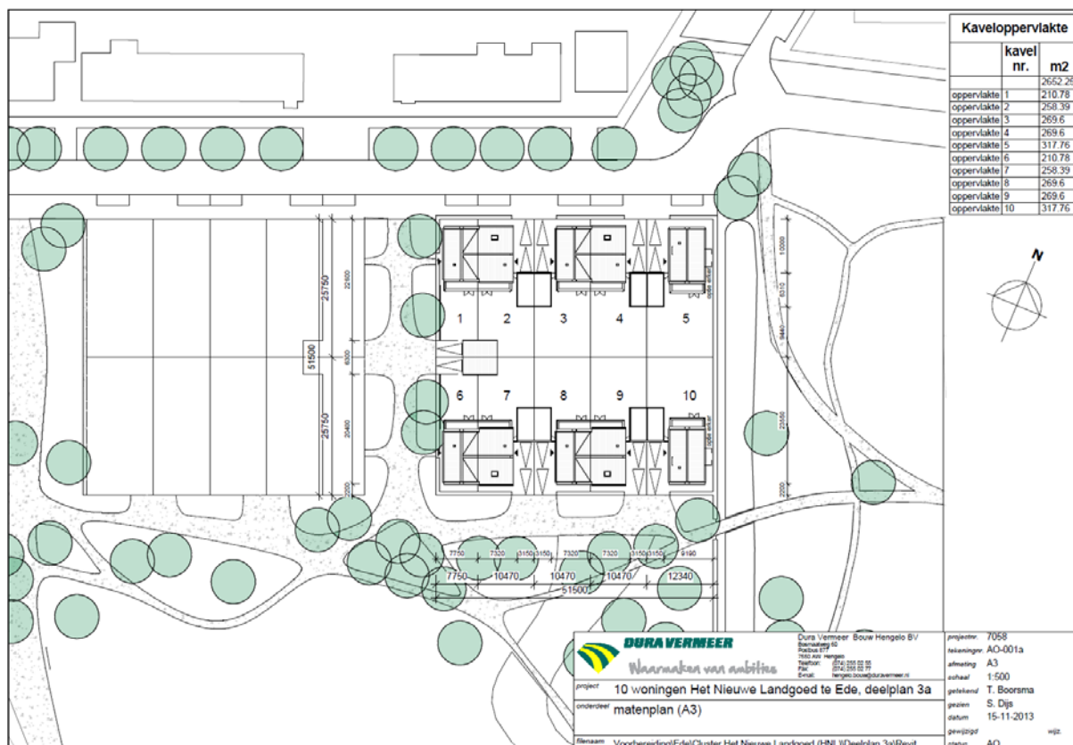
Figuur 1: Matenplan uitwerkingsplan woningen Stakenberg (deelgebied 3a).
