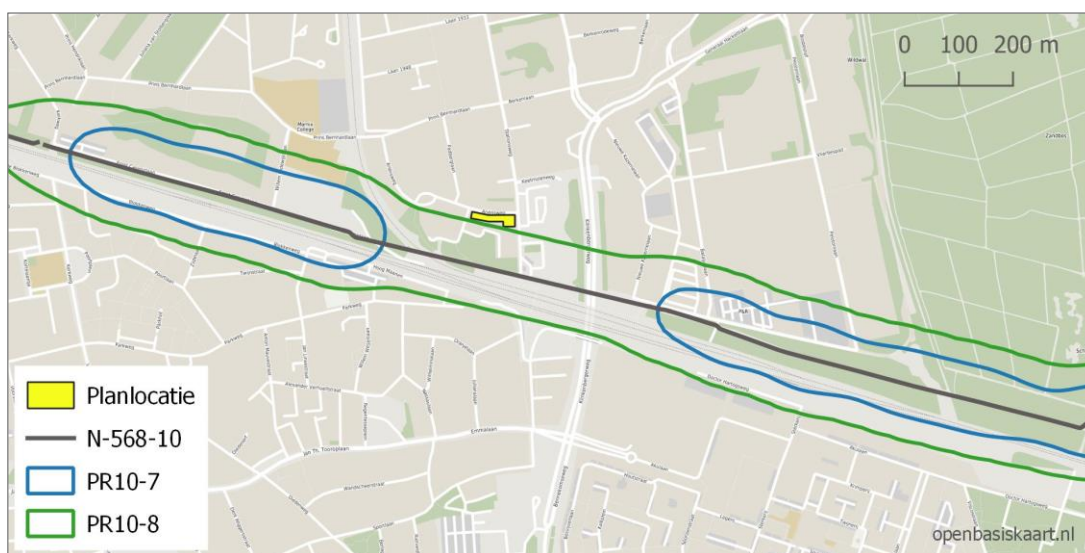
Figuur 2. Plaatsgebonden risicocontouren N-568-10
