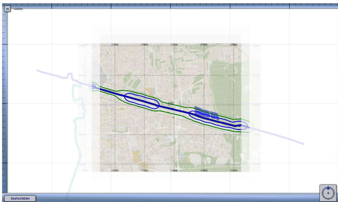
3.1 Figuur 3.1 Plaatsgebonden risico voor 8882_leiding-N-568-10-deel-1 van N.V. Nederlandse Gasunie
