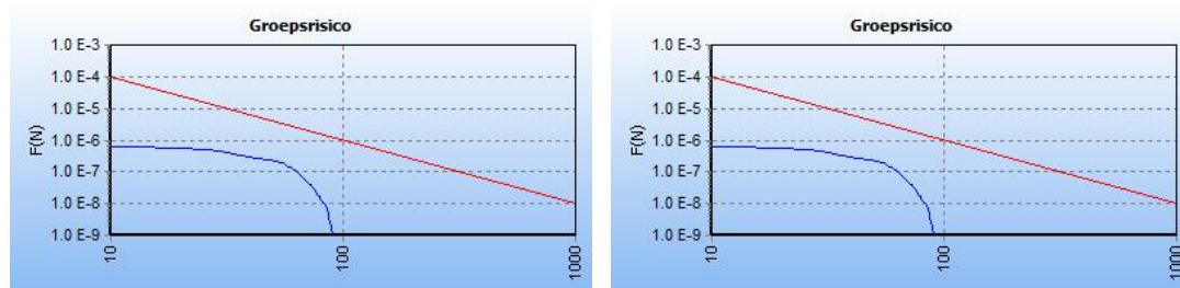
Figuur 3. Groepsrisico N-568-10 huidig (links) en toekomstig (rechts)
