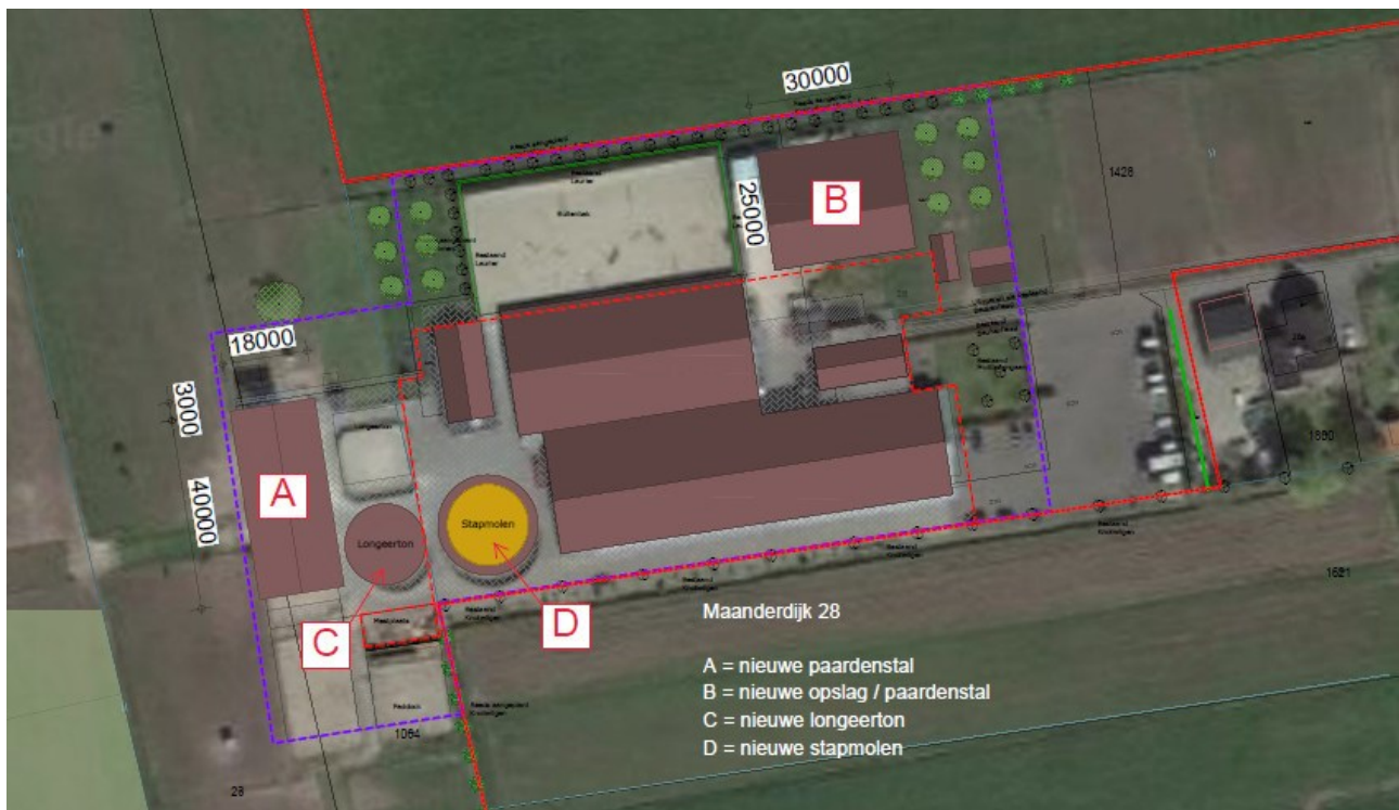
Figuur 3 Situatie (tekening Architect)
