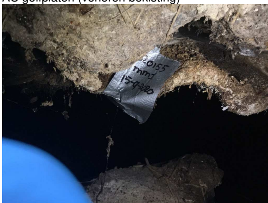
AC golfplaten (verloren bekisting)
