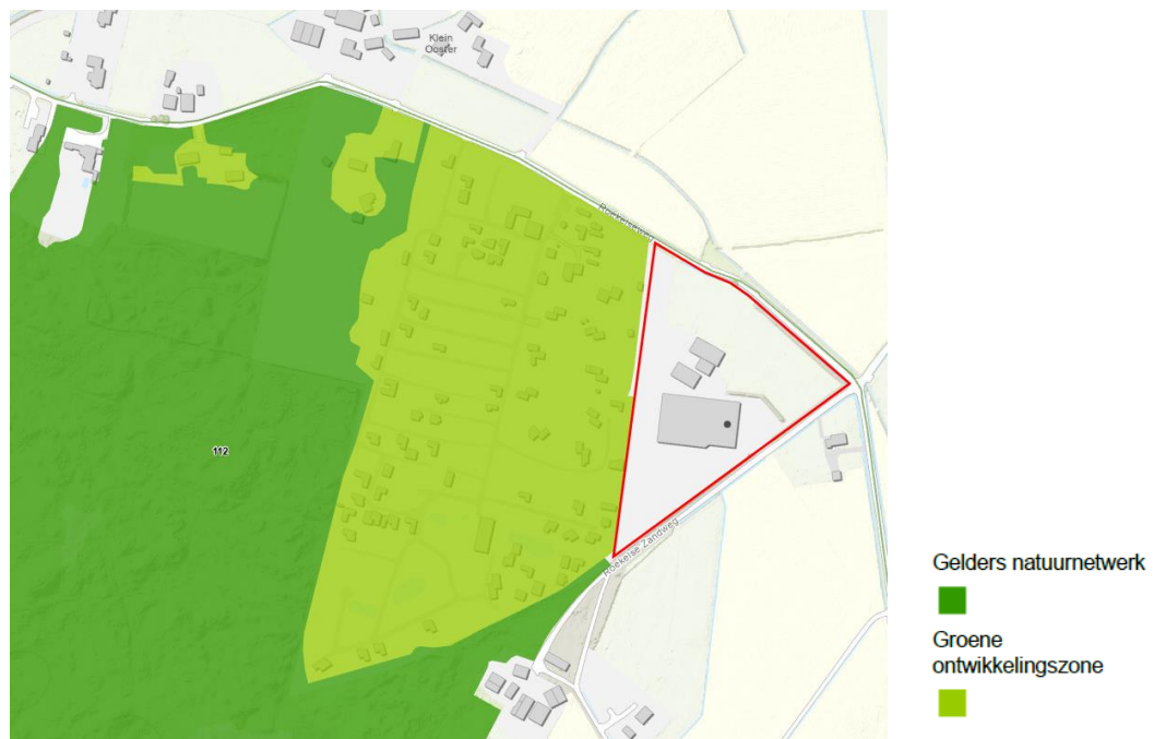
Figuur 15: GNN
