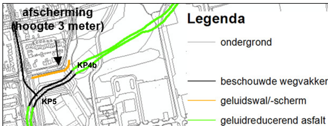
Figuur 3: Overzicht geluidsmaatregelen.
