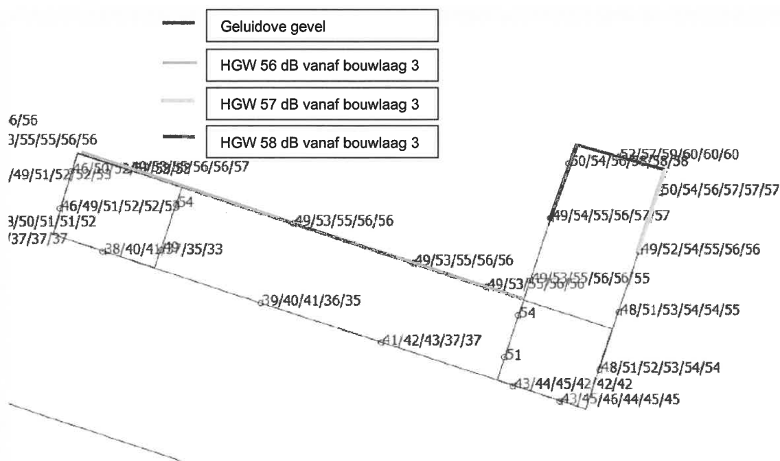
figuur 11: geluidsbelasting gebouw H4 - per bouwlaag
