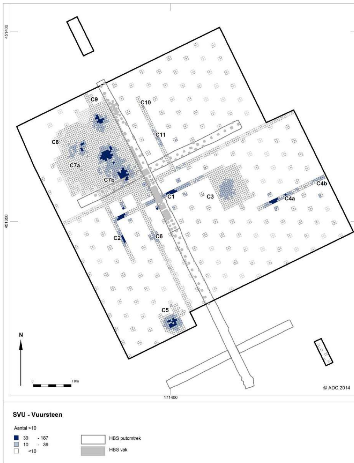
Afb. 7.22 Begrenzing van de vuursteenconcentraties op basis van 10 artefacten per \frac{1}{4} \text{ m}^2 .
