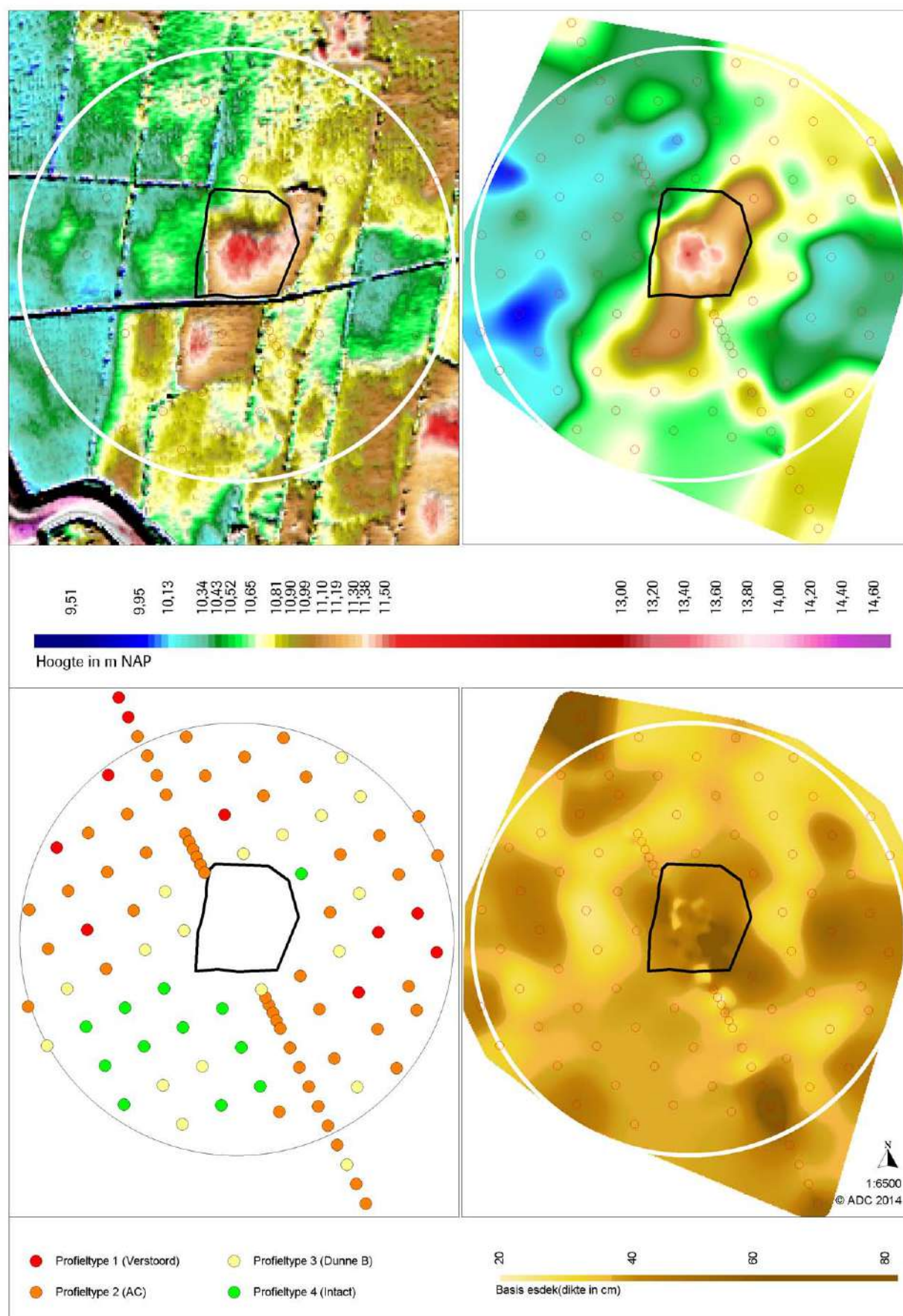
Afb. 3.22 Boorpunten geprojecteerd op het a. AHN en b. paleoreliëf kaart (top zand) en c. profieltypenkaart op basis van de boorgegevens, d. basis van esdek ten opzichte van maaiveld. De reliëfkaarten a en b hebben dezelfde verticale schaal.
