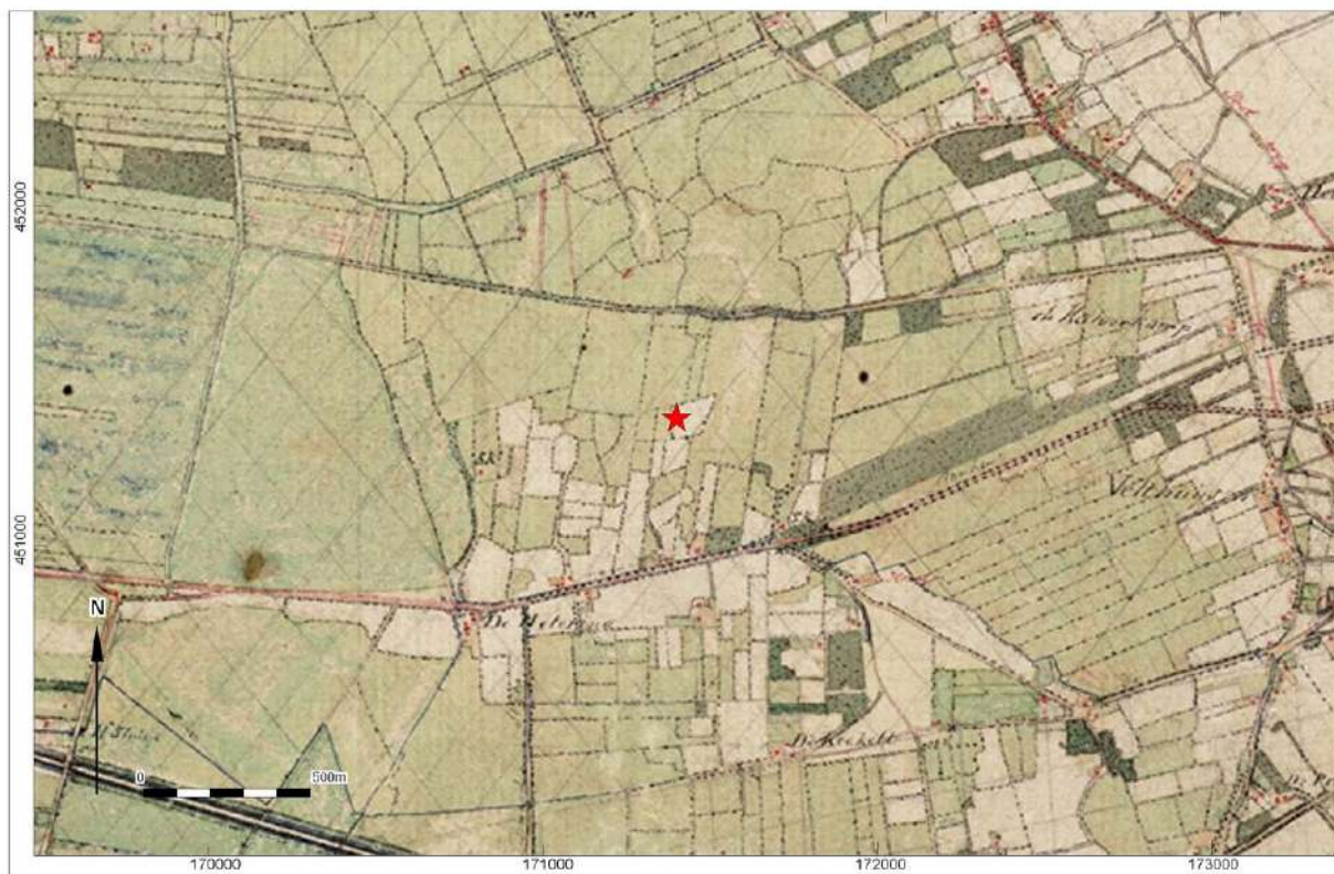
Afb. 3.5 Het onderzoeksgebied (asterix) op het kadastrale minuutplan uit 1832 (Bron: Wolters-Noordhoff Atlasproducties, 1990: Grote Historische Atlas van Nederland, deel 3 Oost-Nederland 1830-1855, Groningen).
