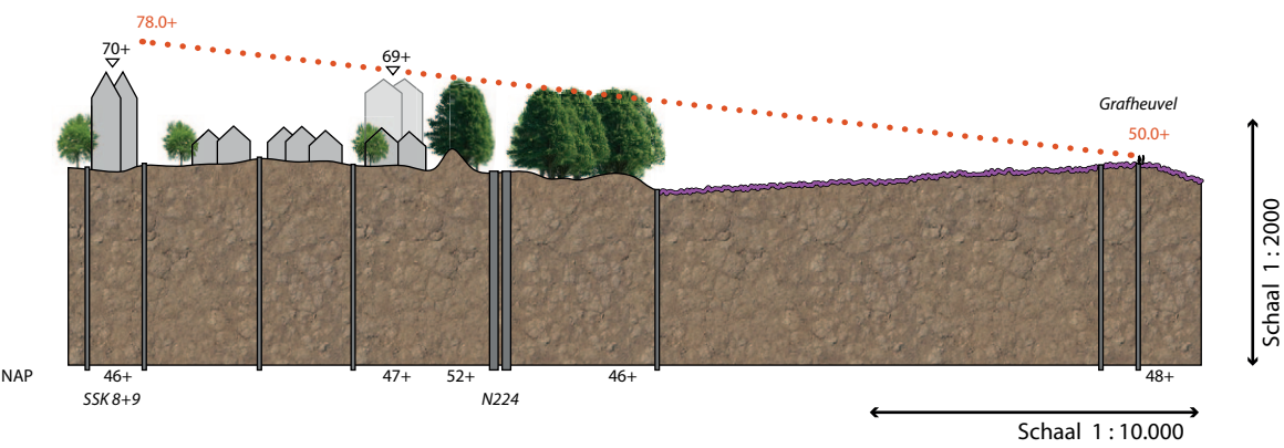
Profiel A-A'
