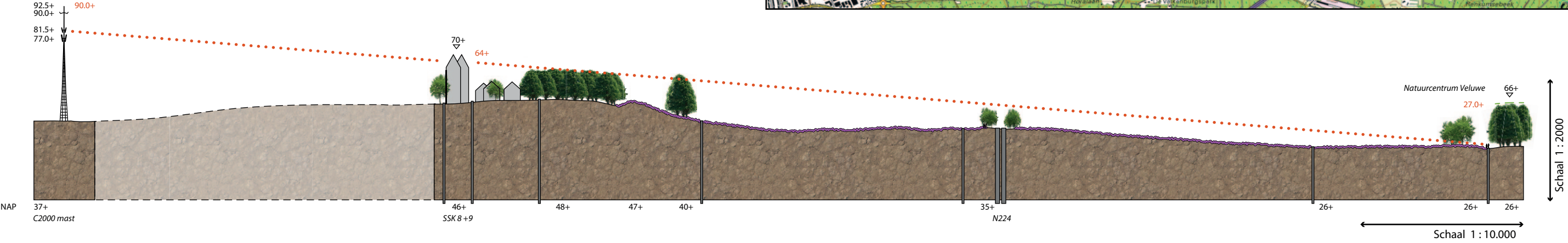
Profiel B-B'
