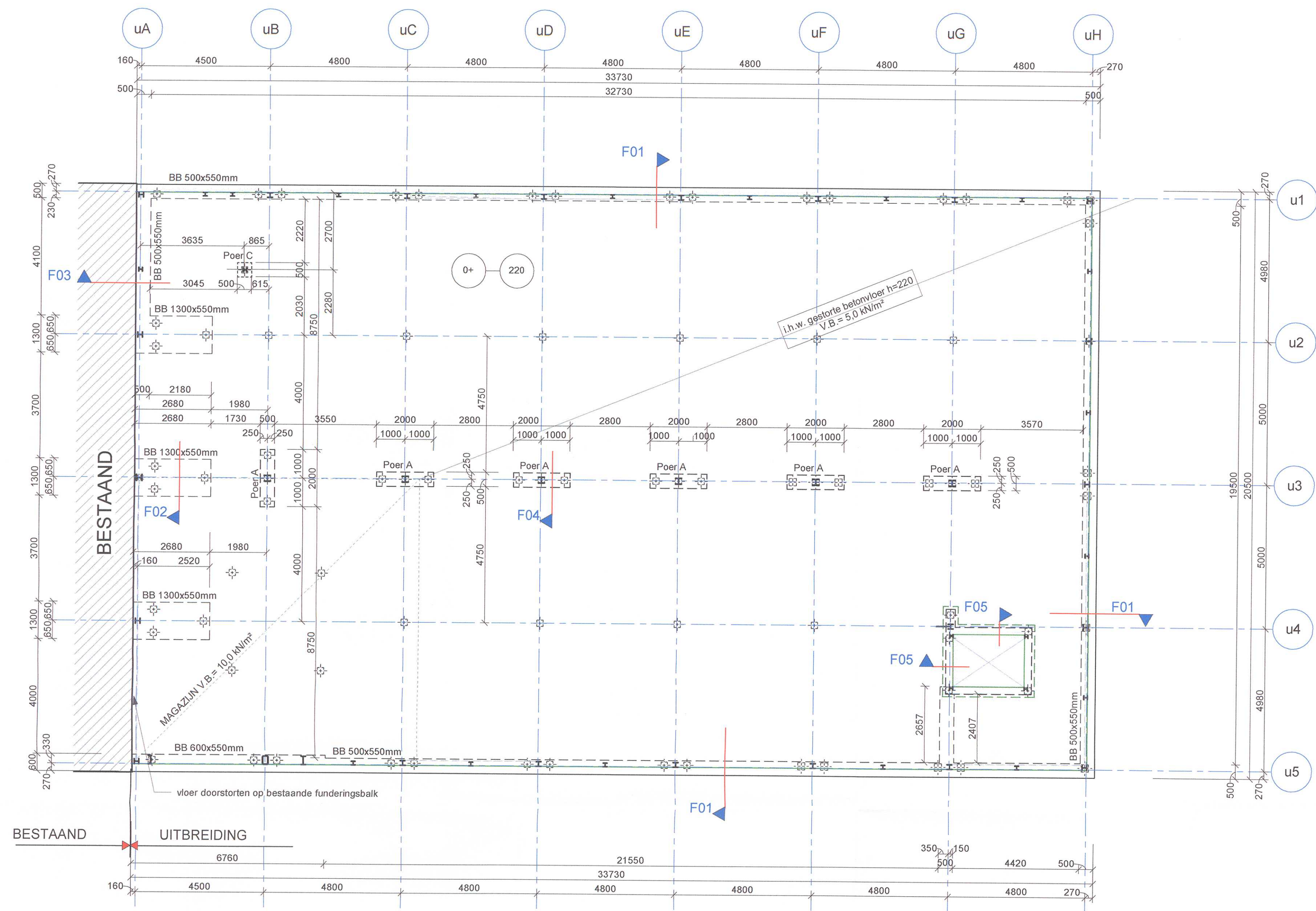
OVERZICHT FUNDERING - BEGANEGRONDVLOER
