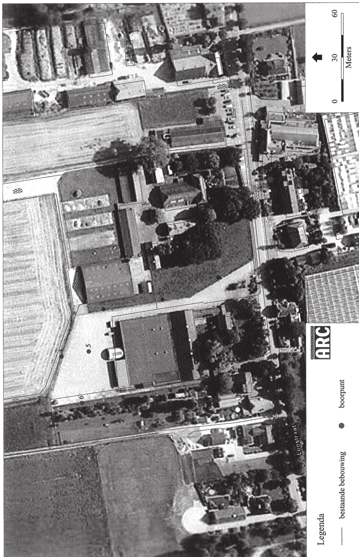
Afbeelding 2 Boorpuntenkaart geprojecteerd op de digitale ondergrond en een luchtfoto van de onderzoekslocatie. Bron luchtfoto: Google Earth.
