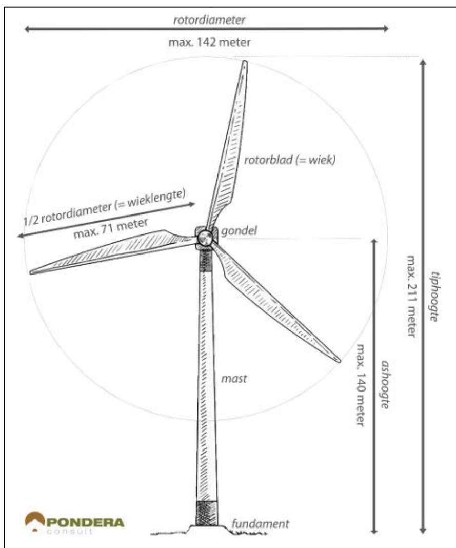
Illustratie windturbine afmetingen en begrippen (Bron: Pondera).
