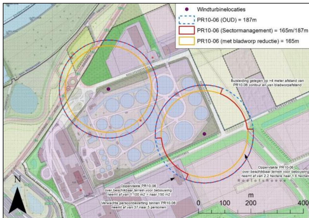
Veiligheidscontouren windturbines, waarbij in rood de veiligheidscontouren bij toepassing van sectormanagement zijn terug te vinden (Bron: Pondera).
