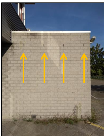
Impressie van open stootvoegen
