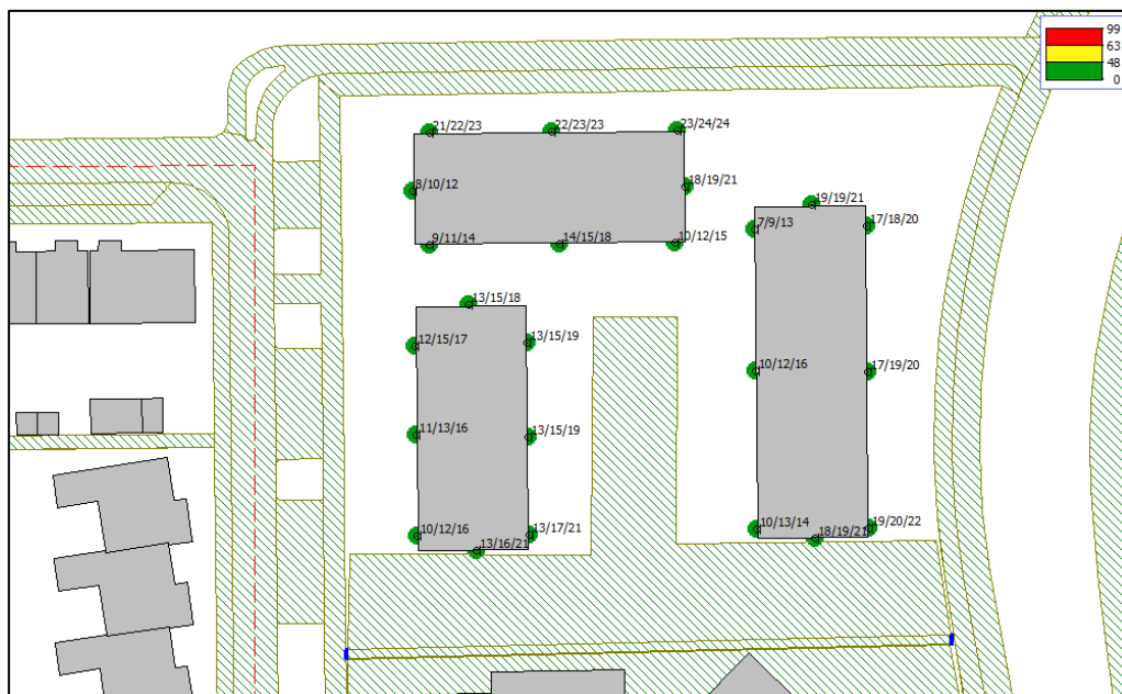
Figuur 6 Geluidbelastingen Golden Delicious (inclusief aftrek art. 110g Wgh)
