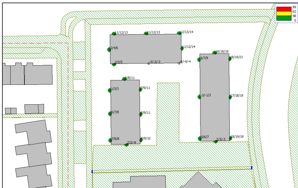
Figuur 7 Geluidsbelastingen Paardenbloem (inclusief aftrek art. 110g Wgh)
