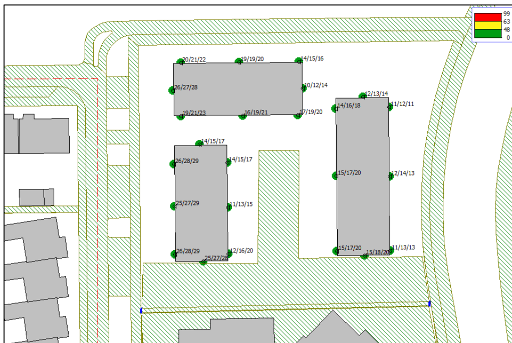
Figuur 4 Geluidsbelastingen Bevelandstraat (inclusief aftrek art. 110g Wgh)
