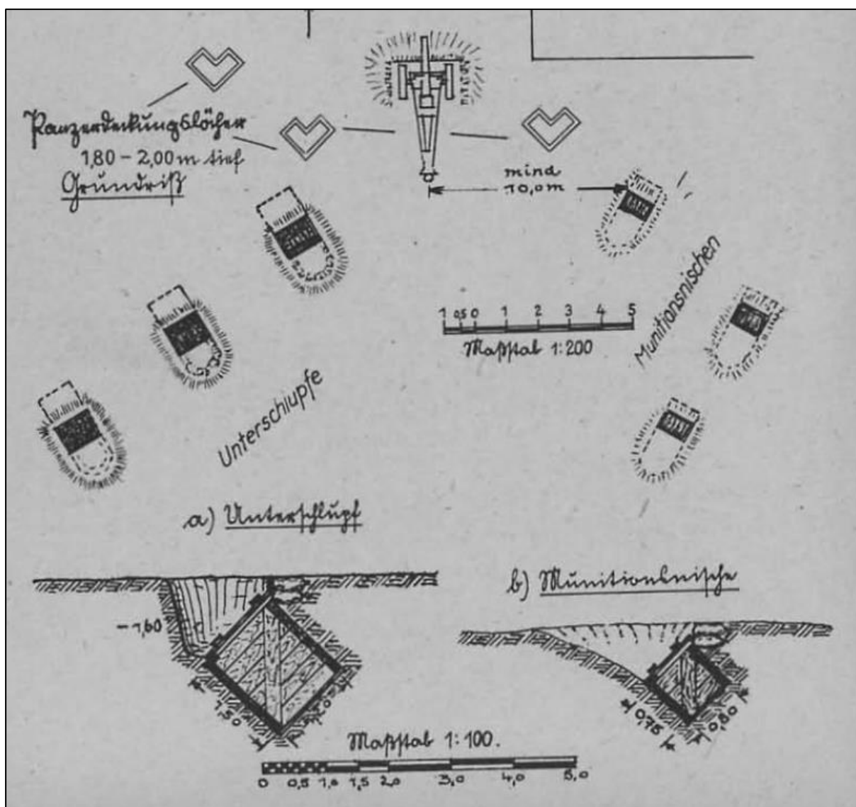
Figuur 23: een schematische weergave van Duitse militaire onderkomens en munitienissen, zoals die rond geschutopstellingen werden aangelegd, zo ook binnen het projectgebied. De minimale afstand tussen het geschut en de munitienissen bedraagt 10 meter. Bron: Bildheft neuzeitlicher Stellungsbau (1 juni 1944).
