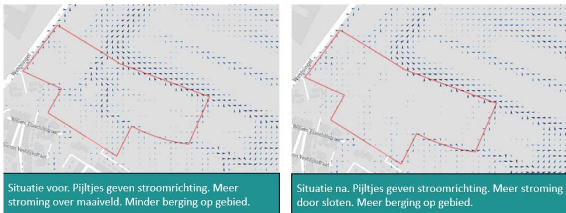
Figuur 5: Stroomrichting afvoer extreme neerslag tijdens piekbui
