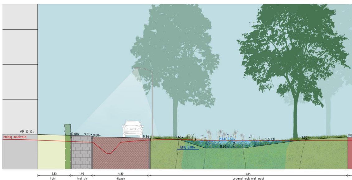
Figuur 8: Wadi's worden dieper gegraven dan het huidige maaiveld, maar niet dieper dan de GHG. (Grond)water wordt niet afgevoerd.
