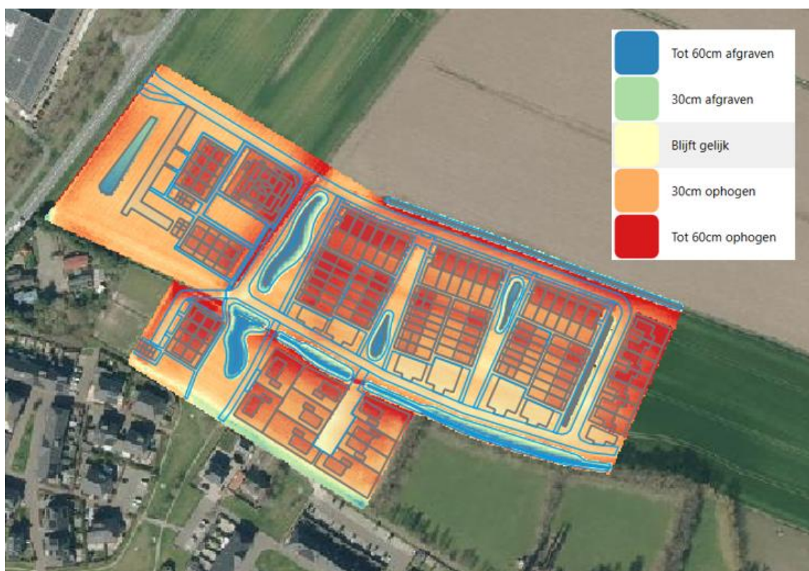
Figuur 4: Geplande aanpassingen maaiveldhoogte en verharding
