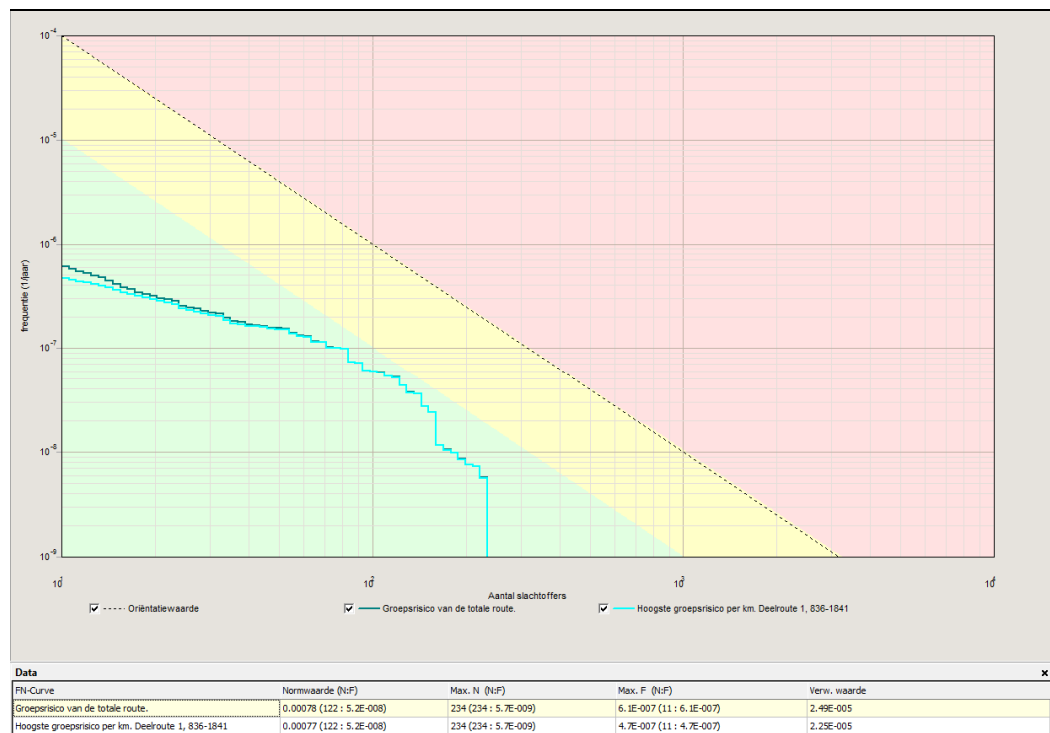
Grafiek 5.2: fN-curve berekend groepsrisico toekomstige situatie
