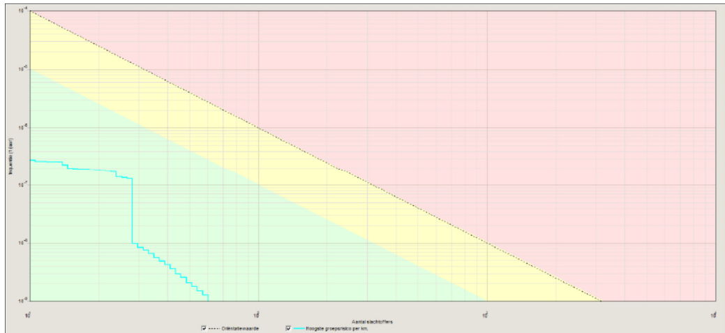
Grafiek 3.1: fN-curve berekend groepsrisico A15
