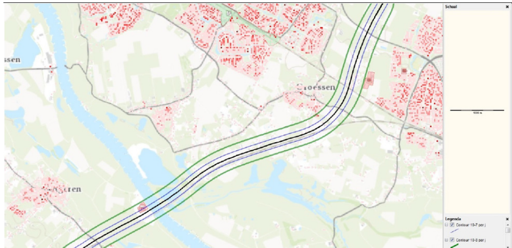
Figuur 3.4: Berekening plaatsgebonden risico traject G100-2 (figuur 35 in rapportage VIA15)
