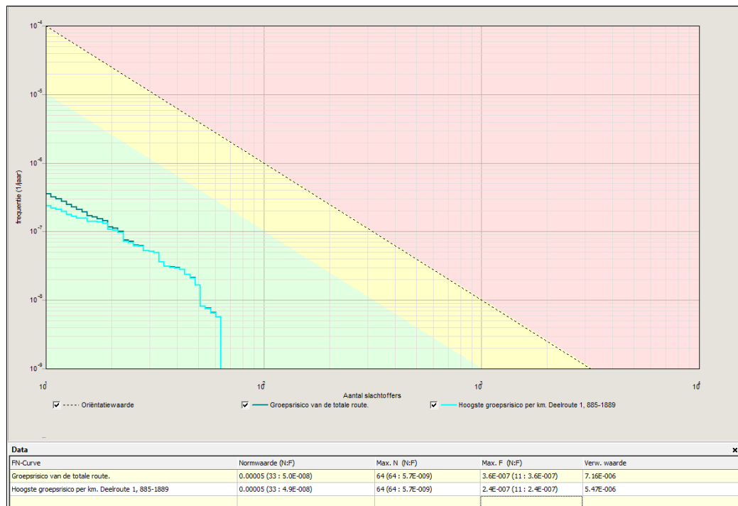
Grafiek 5.1: fN-curve berekend groepsrisico huidige situatie
