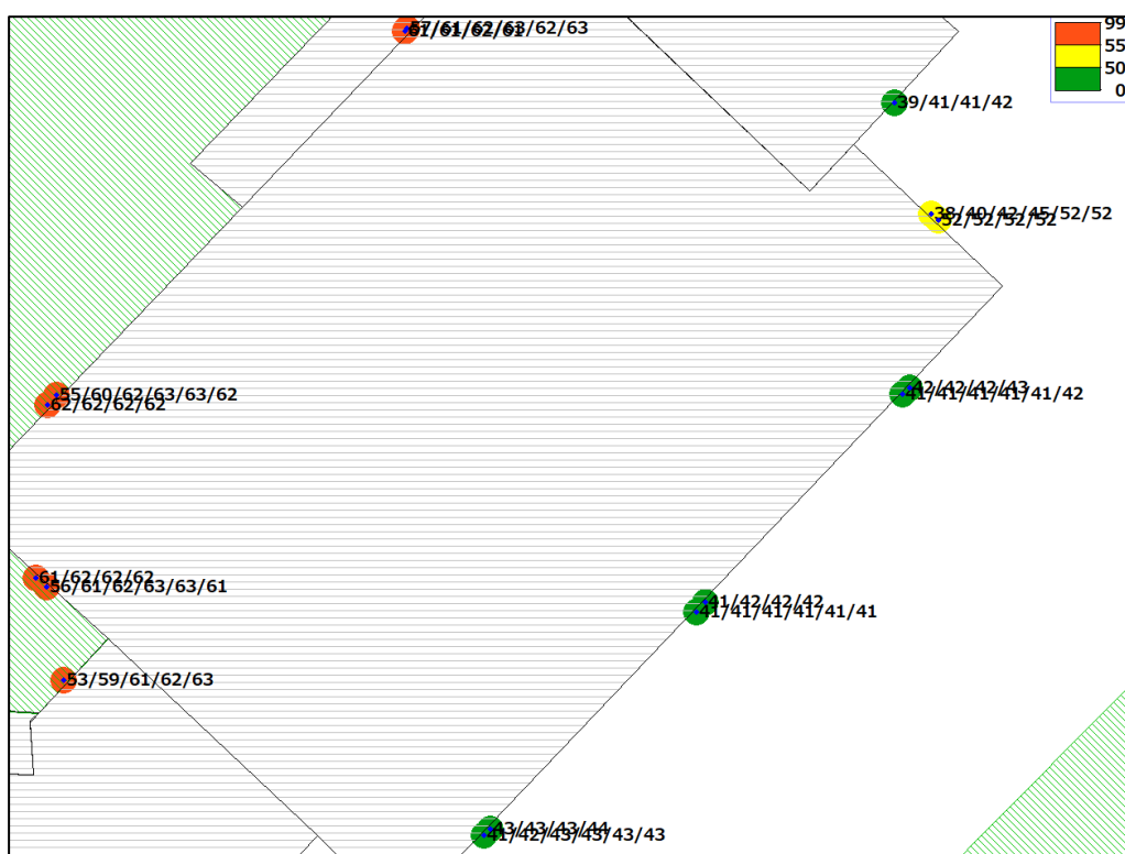
Geluidbelasting in dB(A) 1 e + verdieping gebouw 5, vanwege industrieterrein Hamburgerbroek
