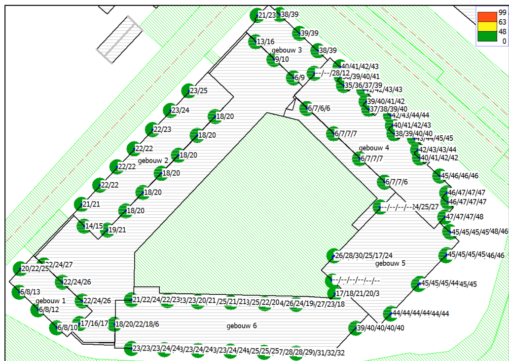
Geluidbelastingen vanaf de 1 e verdieping, vanwege de J.F. Kennedylaan
