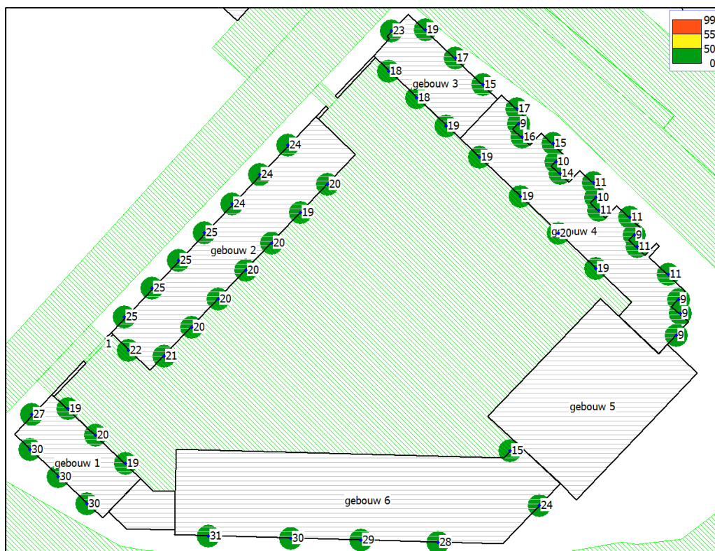
Geluidbelasting in dB(A) op de begane grond, vanwege emplacement Doetinchem
