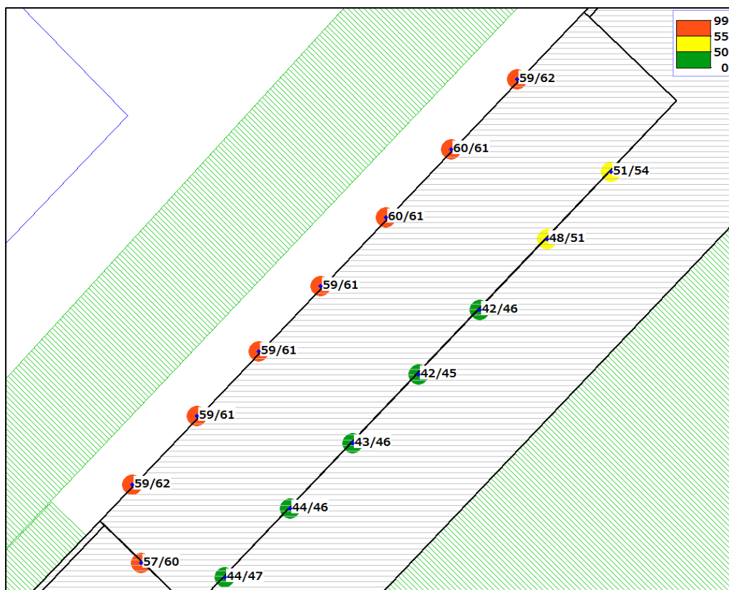
Geluidbelasting in dB(A) 1 e + verdieping gebouw 2, vanwege industrieterrein Hamburgerbroek. De blauwe lijn toont het bebouwingsgebied uit het model van de gemeente.
