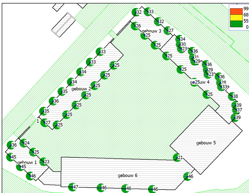
Geluidbelastingen op de begane grond in dB, vanwege de gezoneerde spoorlijnen
