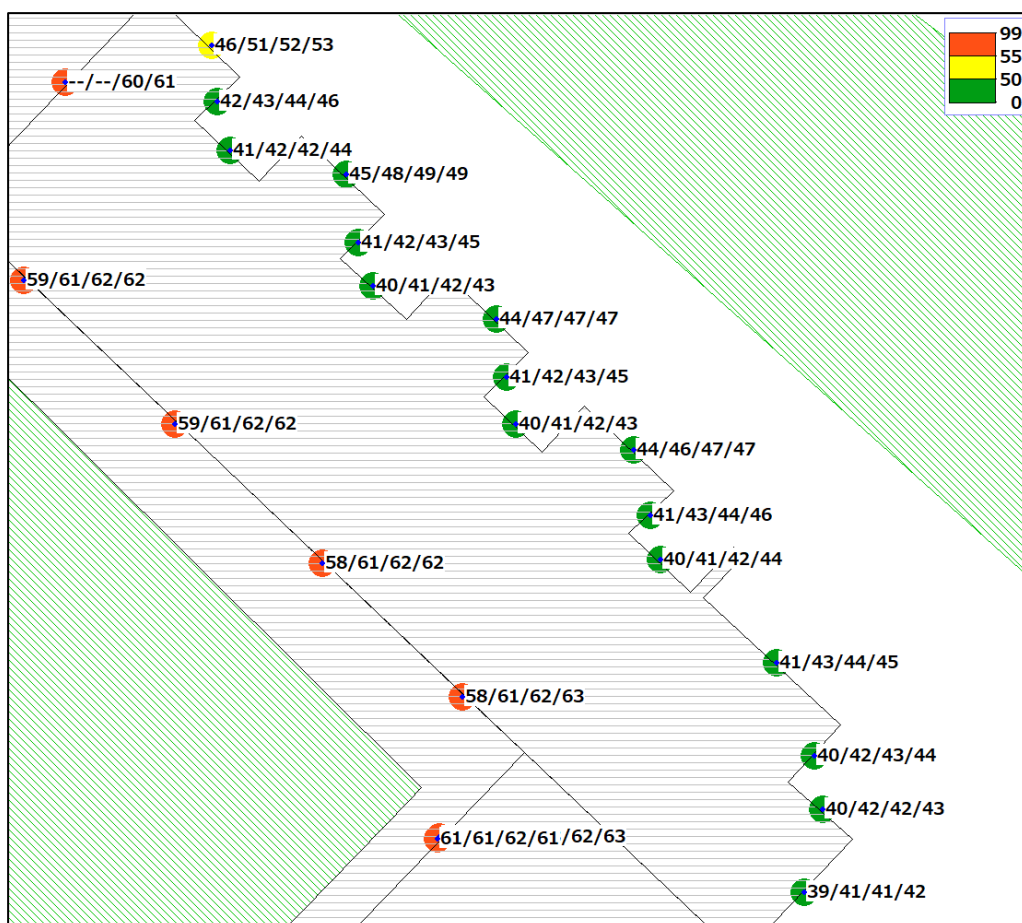
Geluidbelasting in dB(A) 1 e + verdieping gebouw 4, vanwege industrieterrein Hamburgerbroek
