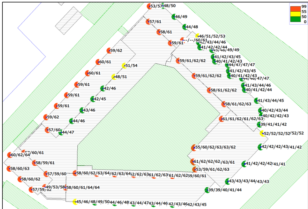
Geluidbelastingen vanaf de 1 e verdieping in dB(A), vanwege industrieterrein Hamburgerbroek, de blauwe lijn indiceert het bebouwingsgebied uit het model van de gemeente
