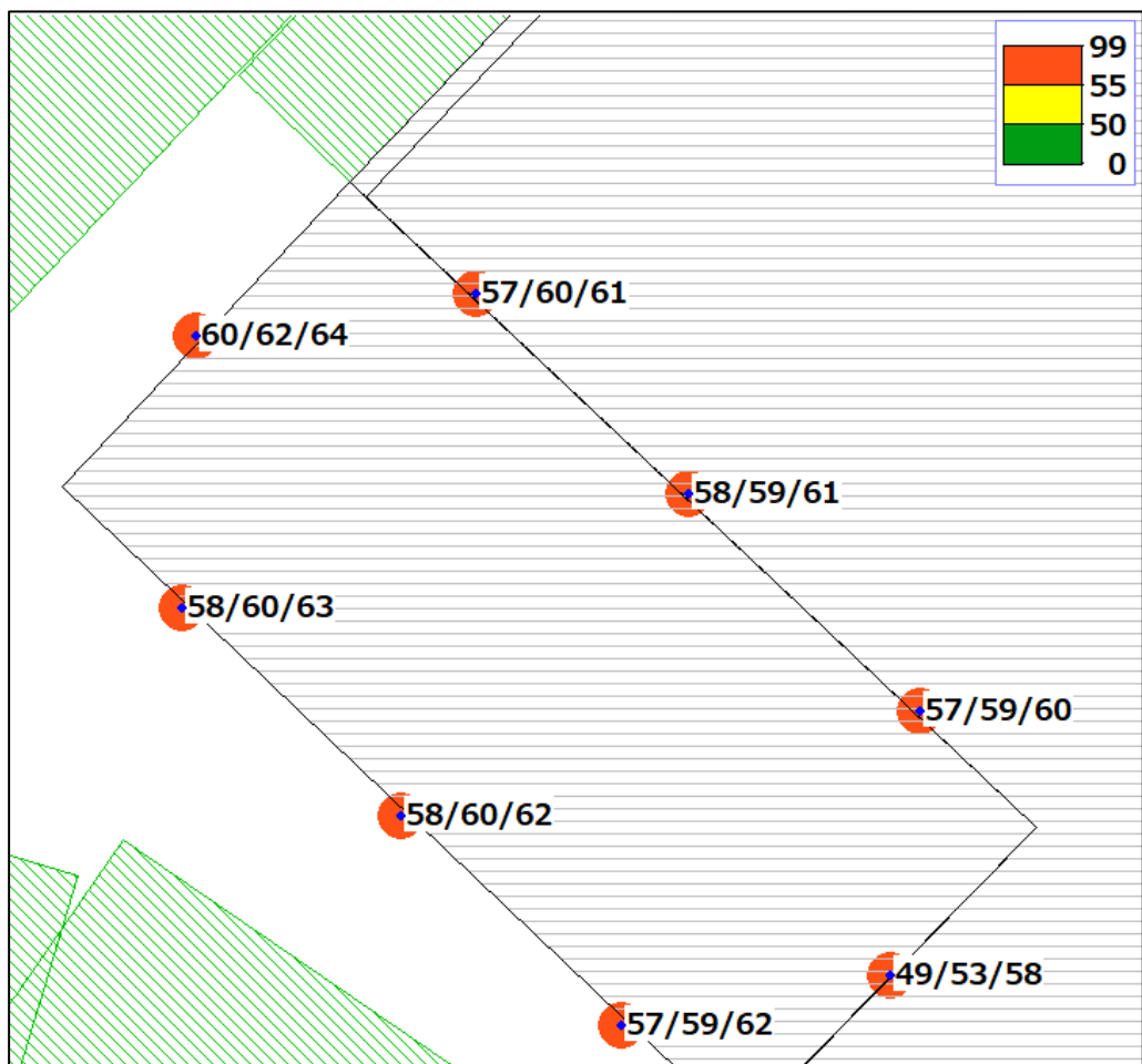
Geluidbelasting in dB(A) 1 e + verdieping gebouw 1, vanwege industrieterrein Hamburgerbroek.
