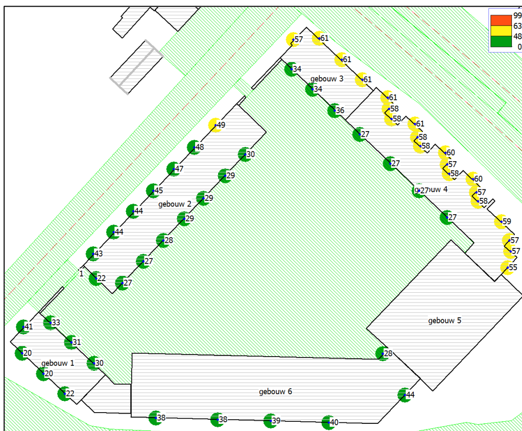
Geluidbelastingen in dB Terborgseweg, van de begane grond.
