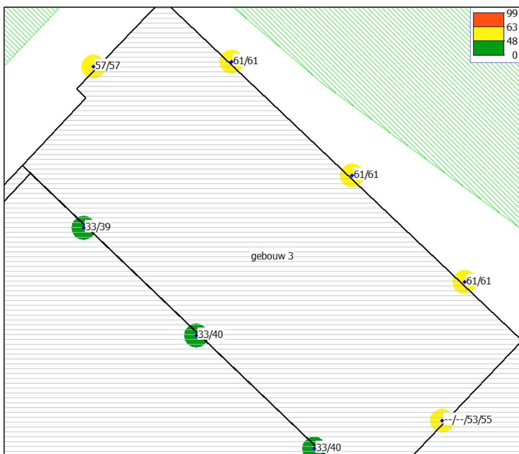
Uitvergroting geluidbelastingen van gebouw 3
