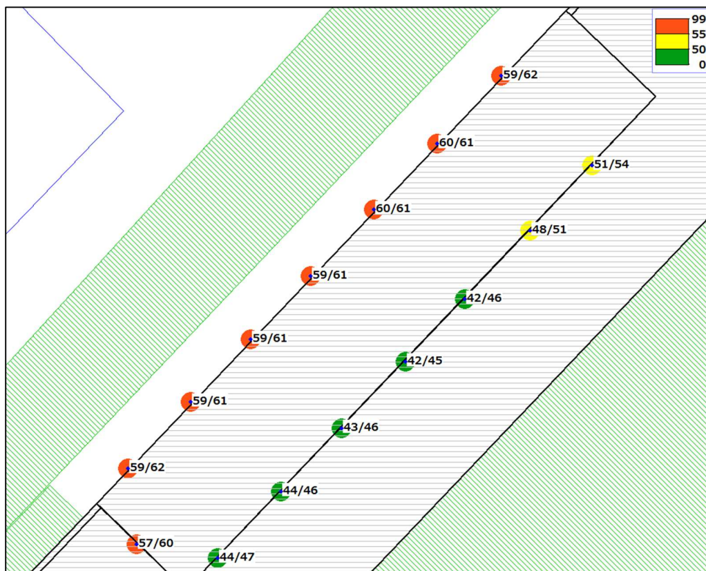
Maatgevende geluidbelastingen gebouw 2, de blauwe arcering betreft het bebouwingsgebied uit het model van de gemeente
