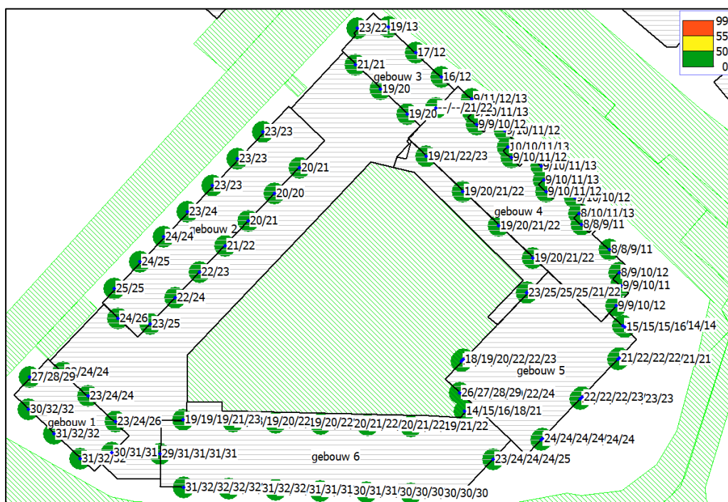
Geluidbelasting in dB(A) vanaf de 1 e verdieping, vanwege het emplacement Doetinchem
