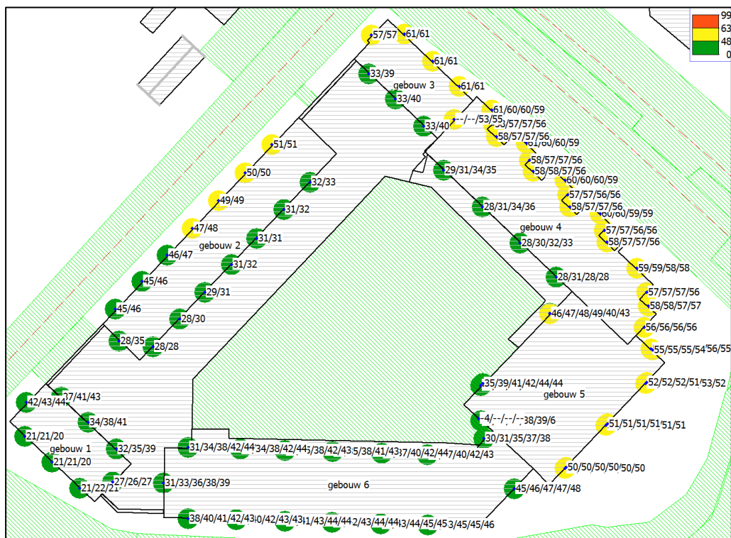
Geluidbelastingen in dB Terborgseweg, vanaf de 1 e verdieping
