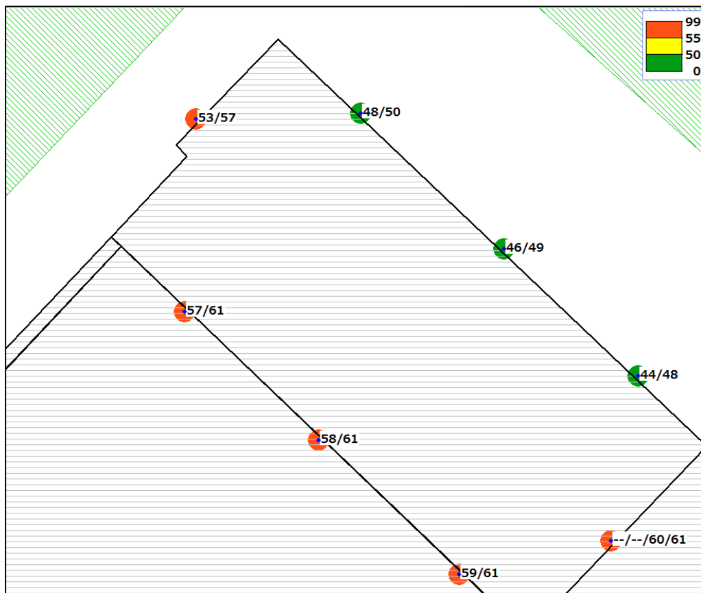
Geluidbelasting in dB(A) 1 e + verdieping gebouw 3, vanwege industrieterrein Hamburgerbroek.
