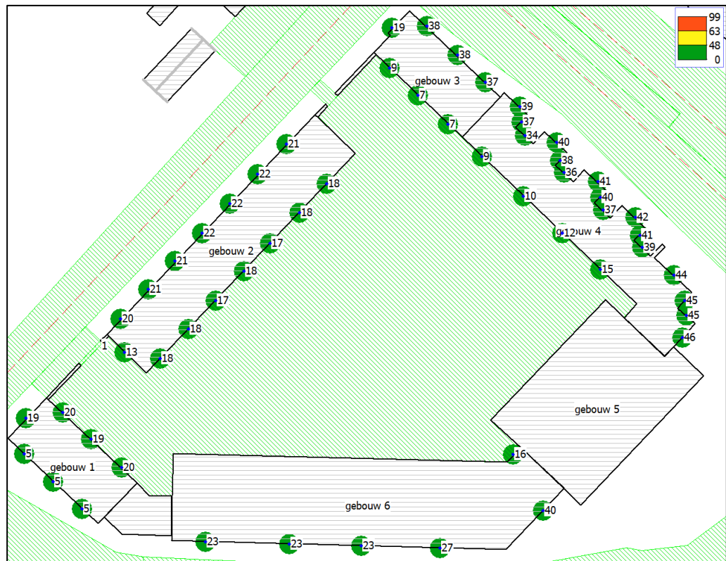
Geluidbelastingen op de begane grond in dB, vanwege de J.F. Kennedylaan
