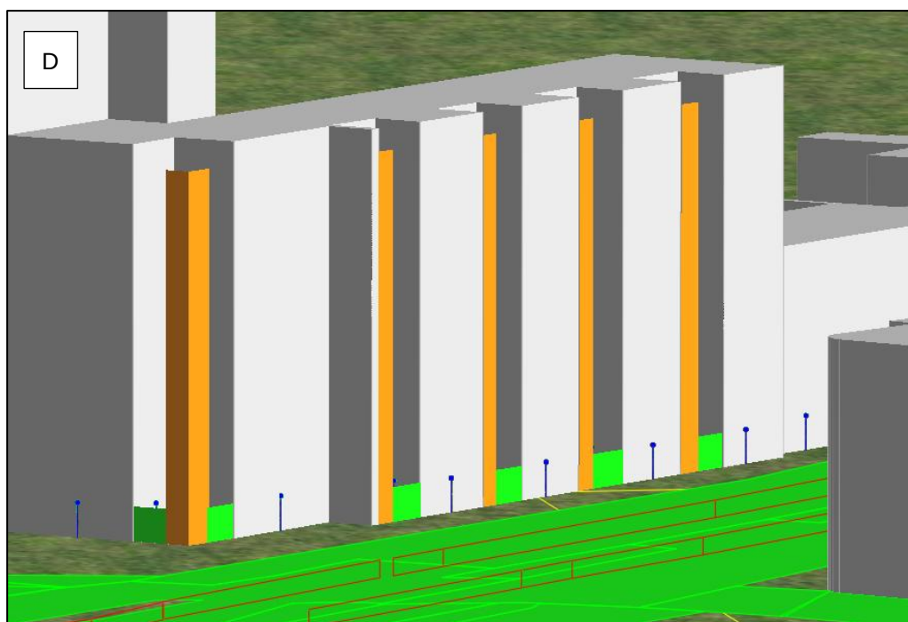
A: twee westelijke woningen gebouw 4; B: 2 middenwoningen gebouw 4; C: de oostelijke hoekwoning van gebouw 4. D: een 3D weergave van de schermen. Aangegeven zijn de verdiepingshoge afscherming (oranje) en schermen van 1,5 meter hoogte (groen) , de minimale lengte van de verdiepingshoge schermen staat boven ieder scherm aangegeven.
