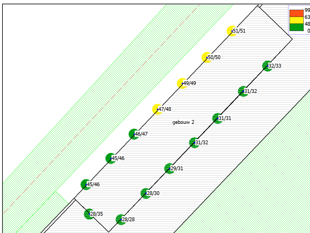
Uitvergroting geluidbelastingen van gebouw 2
