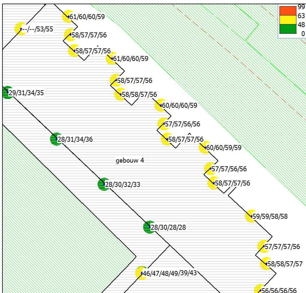
Uitvergroting geluidbelastingen van gebouw 4
