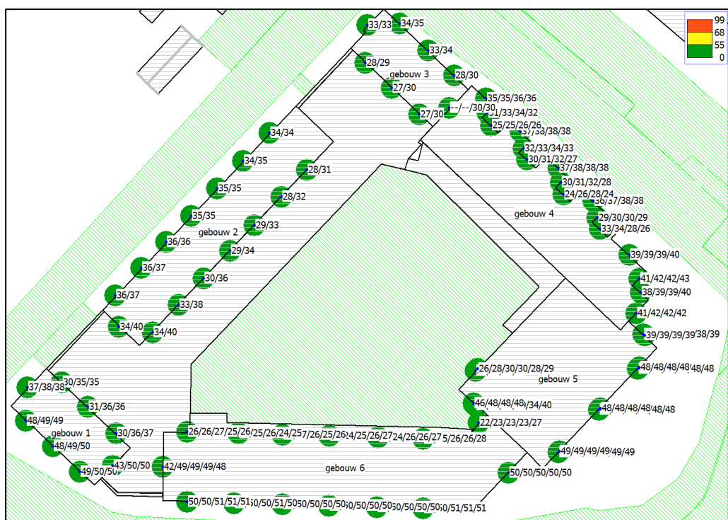
Geluidbelastingen vanaf de 1 e verdieping in dB, vanwege de gezoneerde spoorlijnen
