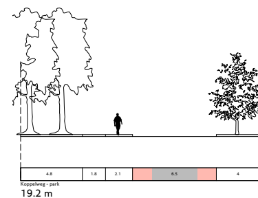
Bestaand profiel
