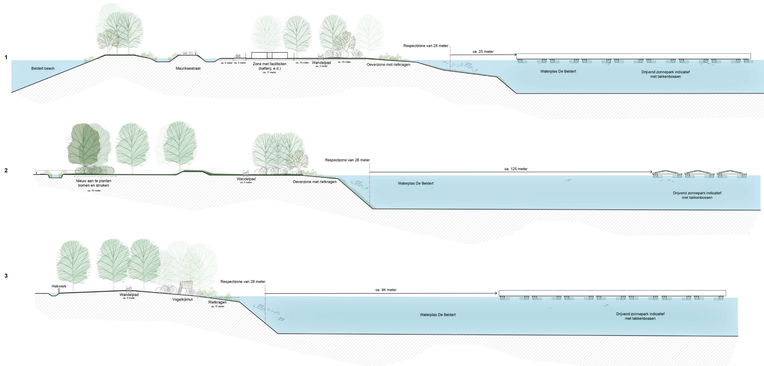
Figuur 11: Dwarsprofielen
