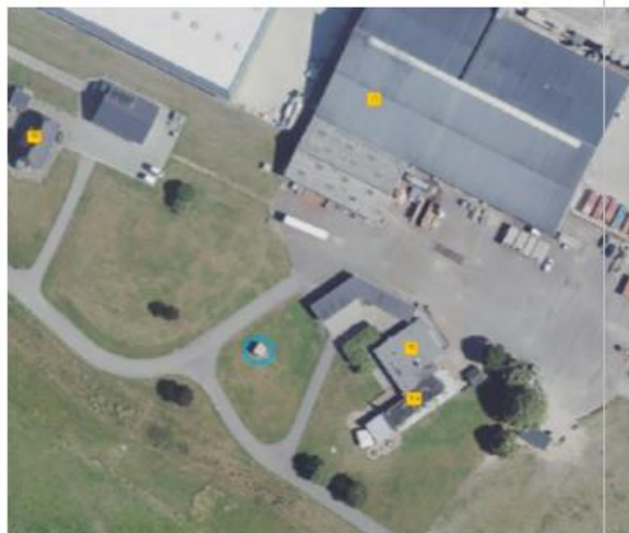
Afbeelding 1b: Locatie van het gasdrukmeet- en regelstation (blauwe cirkel).
