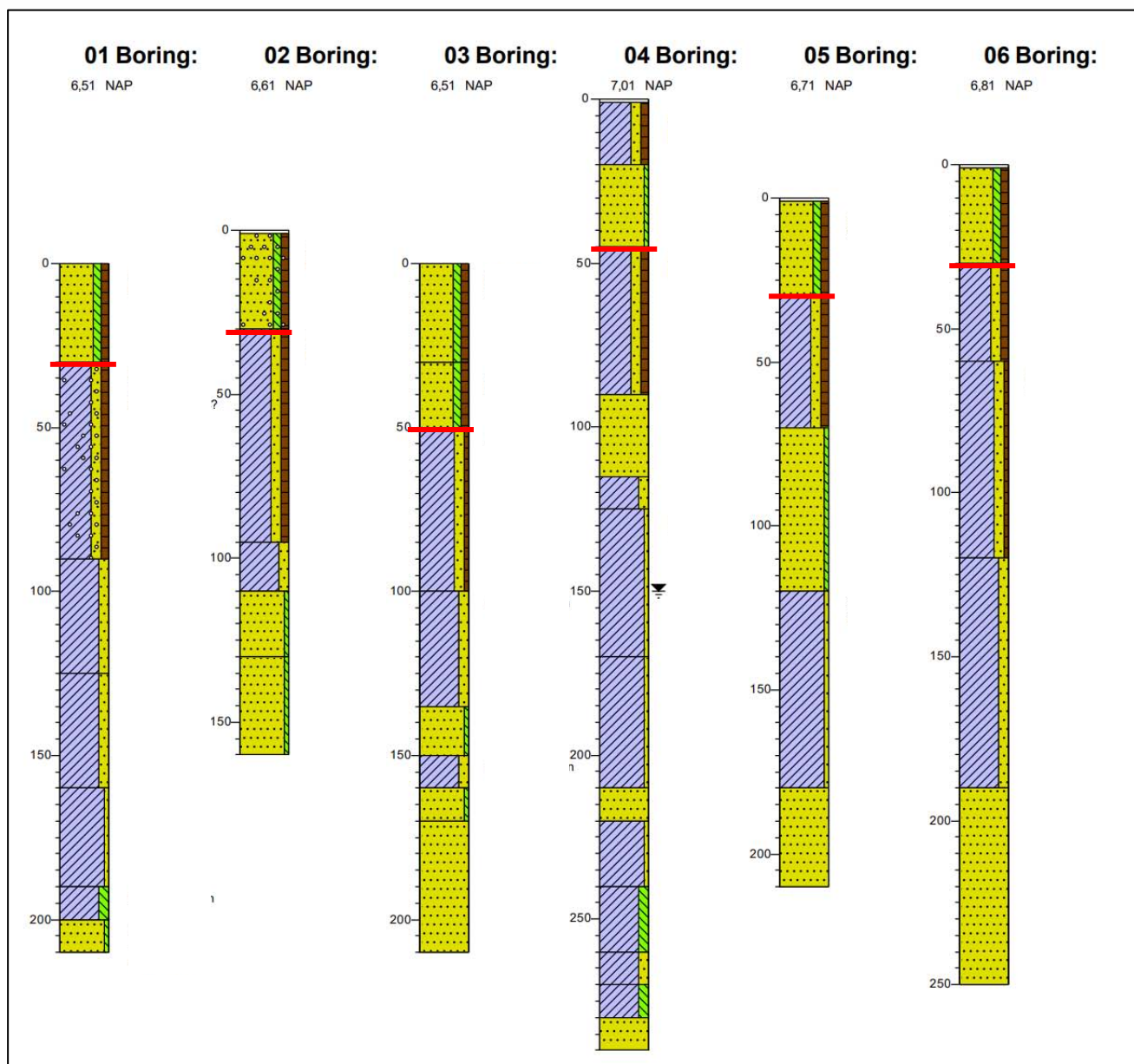
Figuur 7. Overzicht van de boringen, met de hoofdkleuren geel voor zand en blauwpaars voor klei. De bijmengingen zijn weergegeven in groen voor silt en bruin voor humus en grijs voor grind. De rode lijnen geven de grens aan tussen het pakket modern opgebrachte en/of omgewerkte grond en de onderliggende natuurlijke afzettingen. De hoogtes (meter) zijn ten opzichte van NAP.
