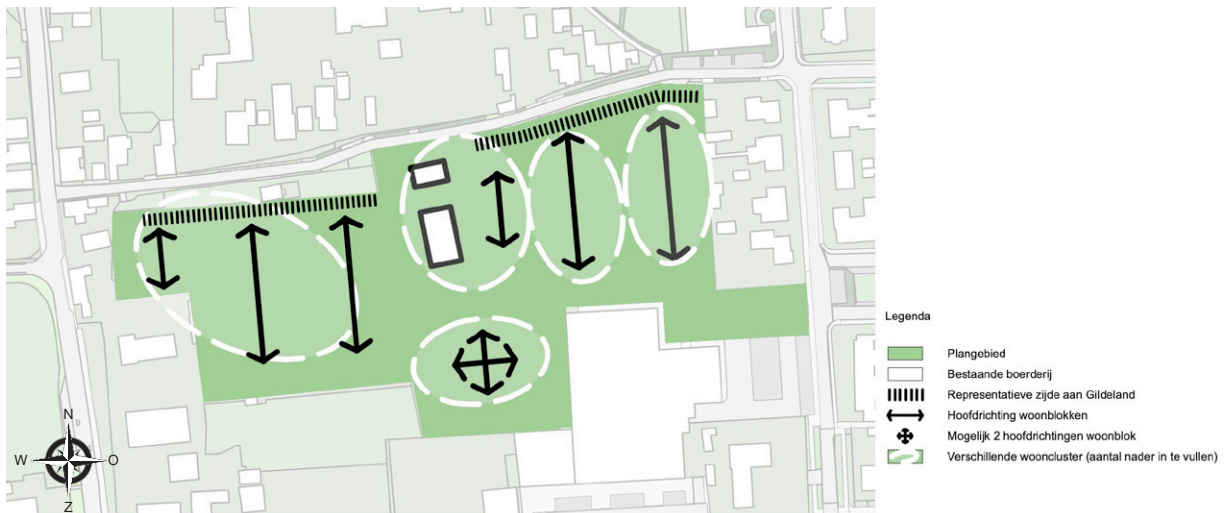
Positionering bouwblokken
