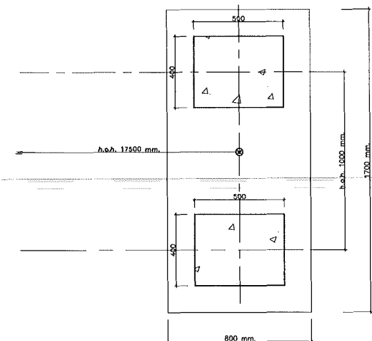
BOVEN AANZICHT FUNDERING Schaaf 1:10
