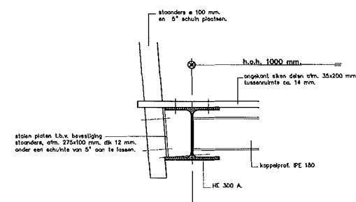
DETAIL D. Schaaf 1:10
