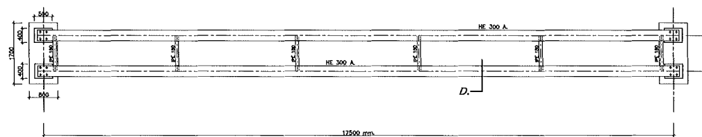
BOVEN AANZICHT staalkonstruktie met fundering
