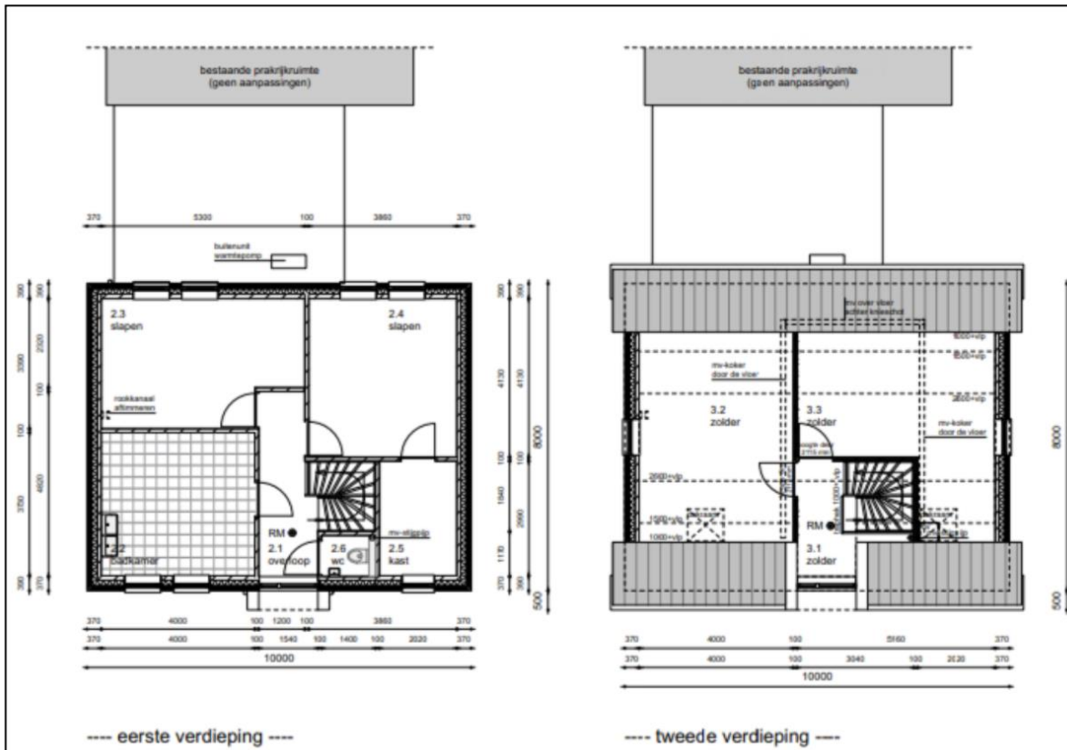
Afbeelding 3.4 Plattegronden eerste en tweede verdieping (Bron: Bouw- en Handelsmaatschappij H.J. Poppink B.V.)
