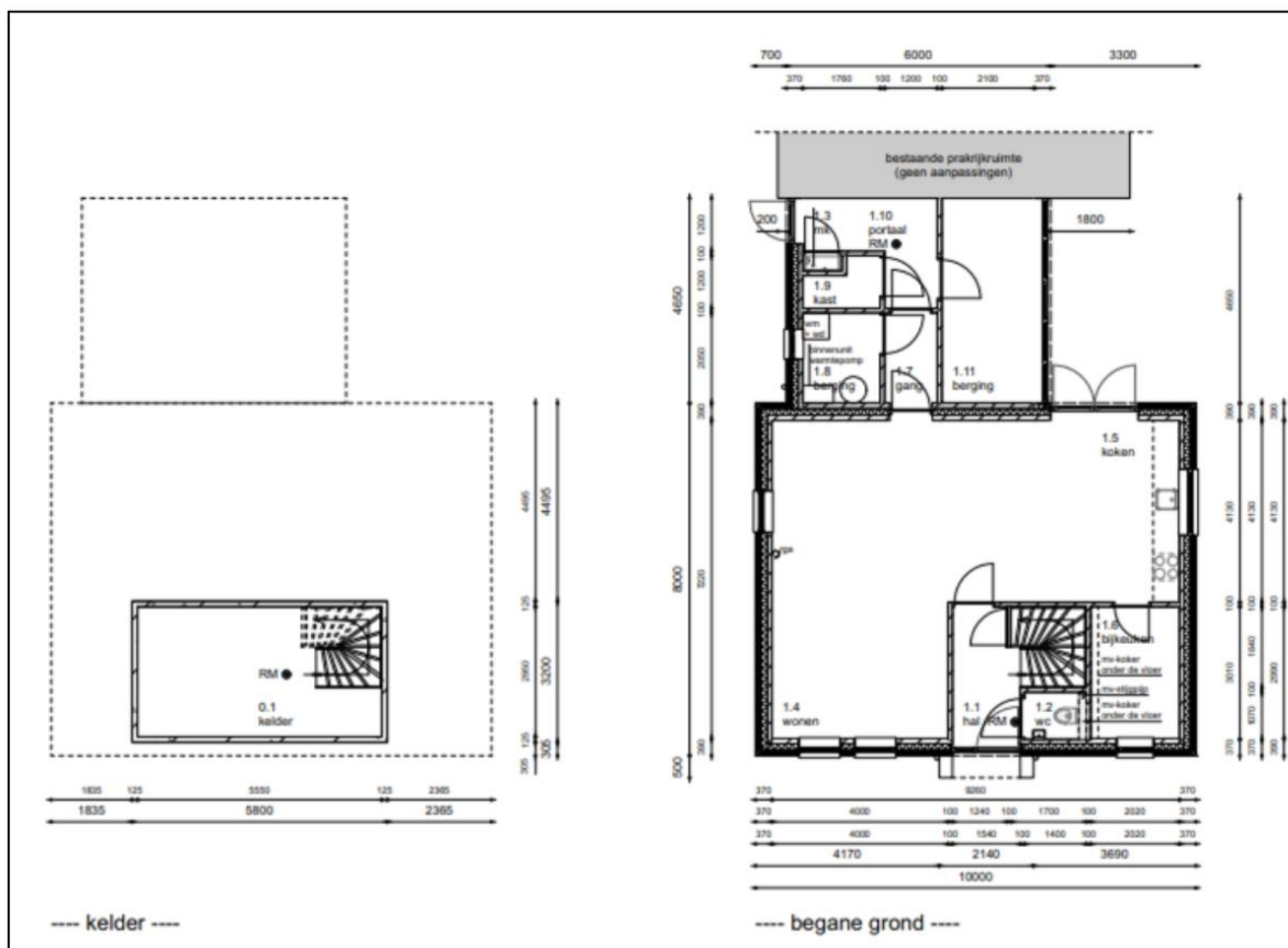
Afbeelding 3.3 Plattegronden kelder en begane grond (Bron: Bouw- en Handelsmaatschappij H.J. Poppink B.V.)
