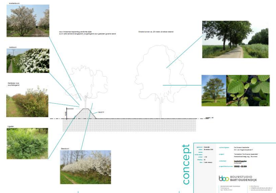
Figuur 7 : Detail grondlichaam Inrichtingsplan (Bron BBO)
