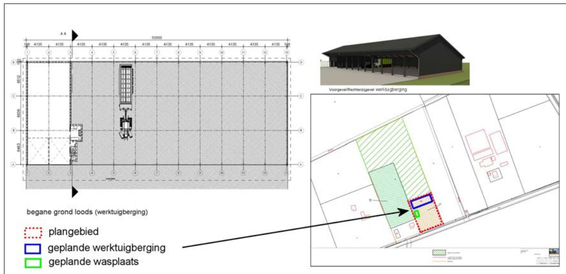
Figuur 2. Hall, Lendeweg 8b: Ontwerpplan voor de werktuigberg en de wasplaats (bron: Bonekamp Advies bv, Twello; zie ook Appendix IV).
