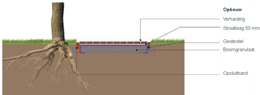
Fig. 25. Schematische weergave opbouw cunet.
