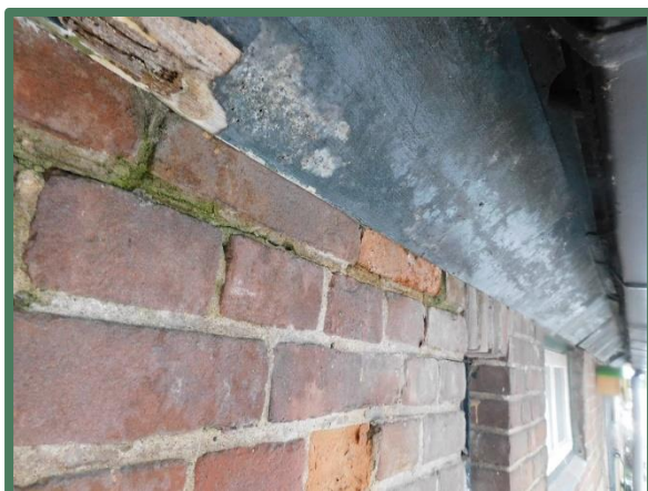
Aansluitend boeiboord
