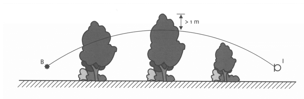
figuur 3.10 Het gekromde geluidspad gaat door twee 'regels' vegetatie
