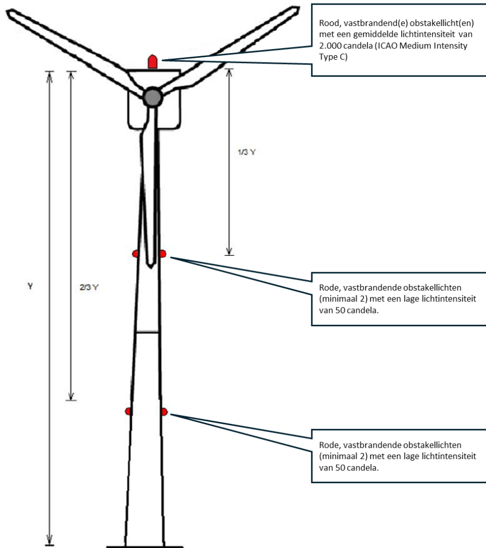
Figuur 4 Principetekening obstakelverlichting bij schemerlicht en nacht met tiphoogte groter dan 210 meter.
