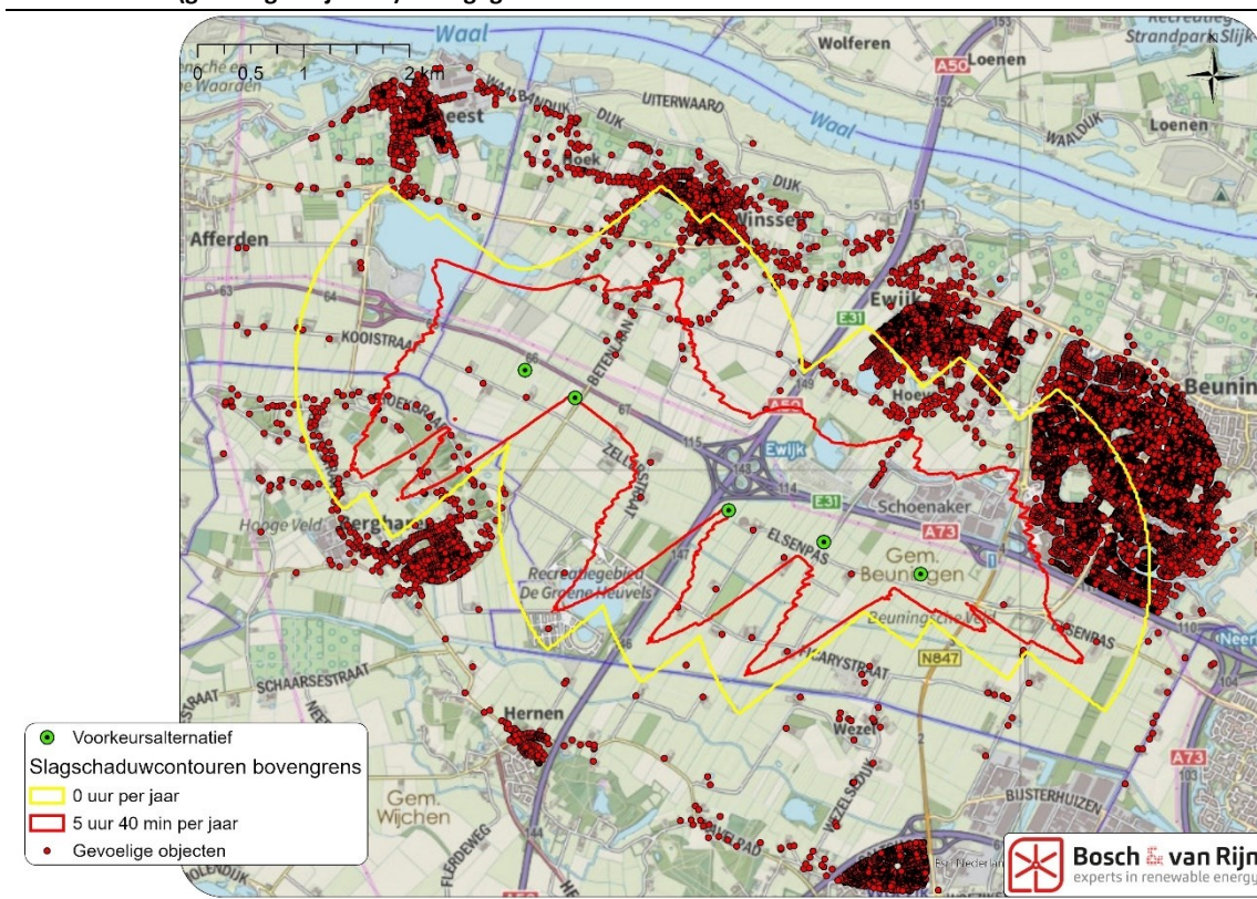
Figuur 12 De 5:40u en 0u slagschaduwcontouren van de bovengrens. Hierbij zijn ook nabijgelegen woningen (gevoelige objecten) weergegeven.
