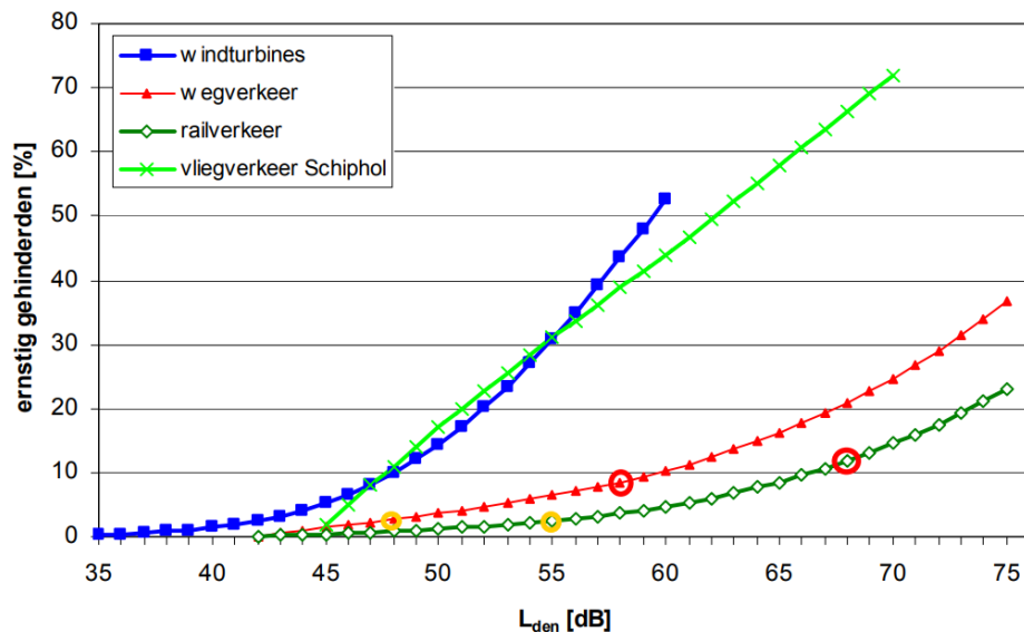
Figuur 7 Relatie tussen Lden en het percentage ernstig gehinderden (binnenshuis) bij verschillende bronnen (Verheijen, et al., 2009). Bij 47 dB Lden geluidsbelasting van windturbines (blauwe lijn) hoort een ernstig-gehinderdenpercentage van ca. 9%. De normen voor railverkeer (68 dB Lden) en wegverkeer (58 dB Lden) zijn met rode cirkels weergegeven en leiden tot vergelijkbare hinderpercentages.
