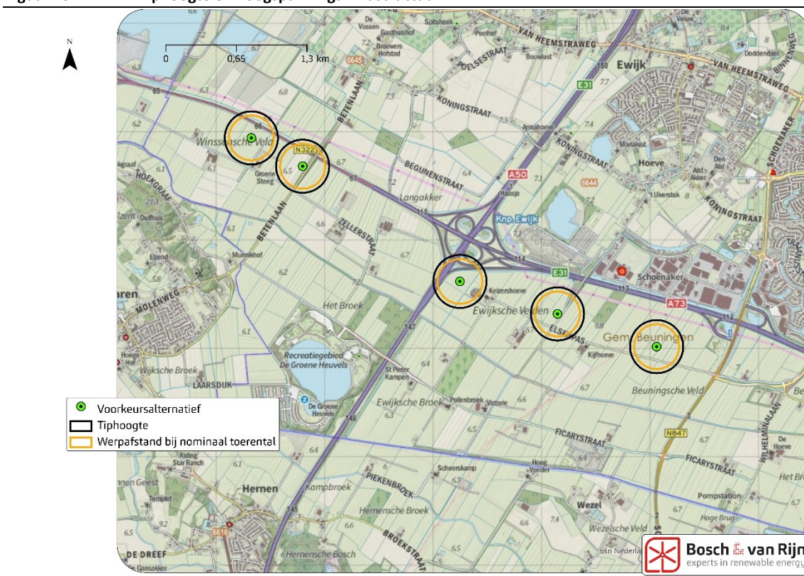
Figuur 19 Tiphoogte en hoogspanningsinfrastructuur
