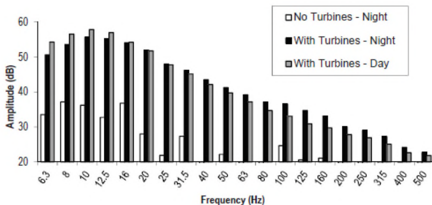
Figuur 2 Data van LfG (dB) gemeten in de betreffende slaapkamer van een huis in de buurt van een windmolen (Alves-Pereira, and Castelo Branco, 2014).
