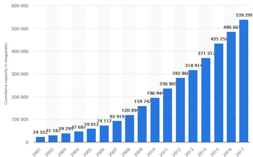
Figuur 1 Ontwikkeling cumulatief geïnstalleerd vermogen aan windenergie in de wereld tussen 2001 en 2017 ( www.statista.com , 2018).
