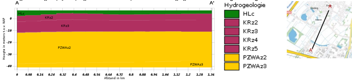
Figuur 1: Geohydrologisch model gebaseerd op REGIS II.1 (bron 3C)
