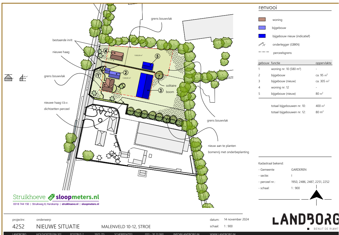
Afbeelding 1.4: Nieuwe situatie. Bron: 4252, overzicht slopen, Malenveld 8-10-12, Stroe, 2023.
