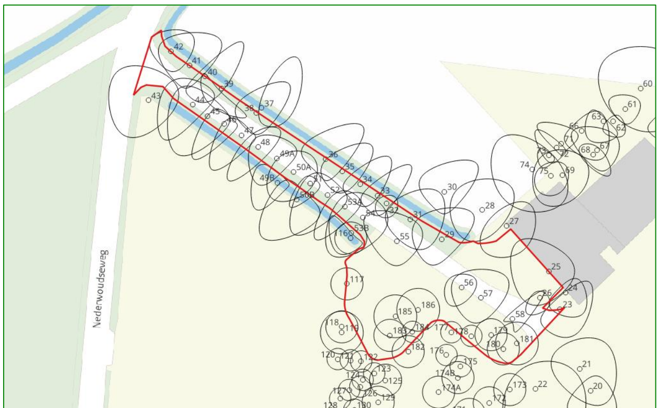
Figuur 9: Ontgravingscontour asbestsanering
